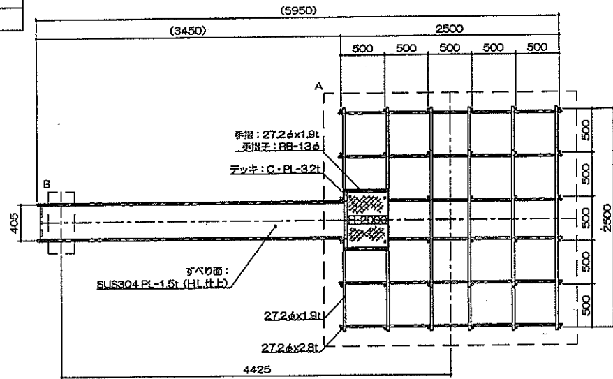
各階組立平面図 S=1:100
