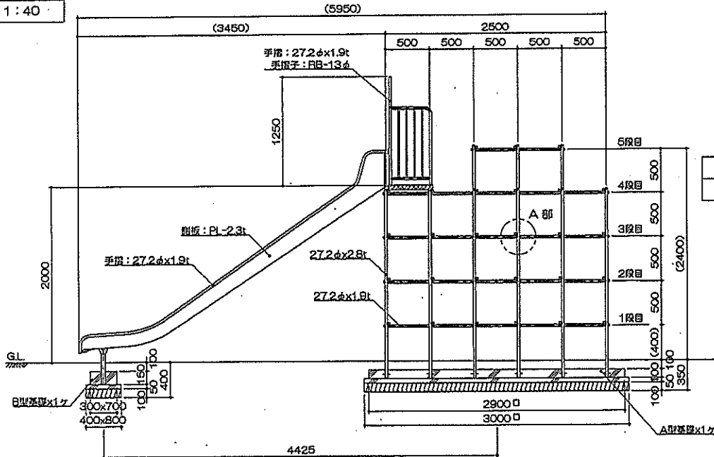
立面図 S=1:40
