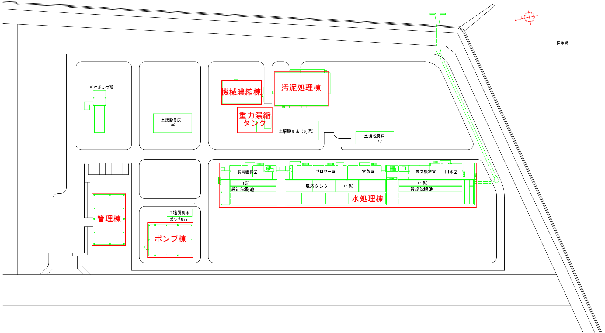
福山市下水道総合地震対策計画 松永浄化センター対象施設配置図
