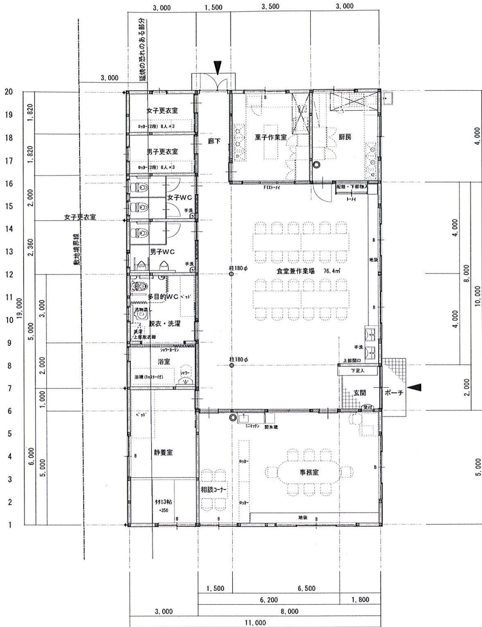
平面図 S=1:100
