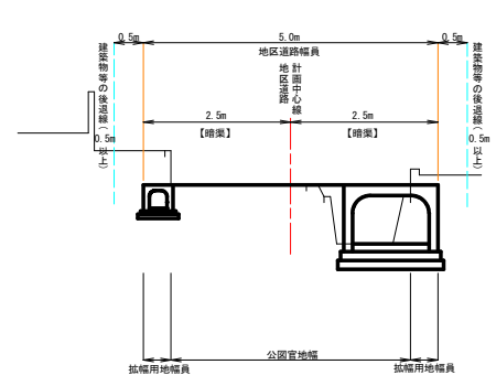
標準断面図 S-1-50
