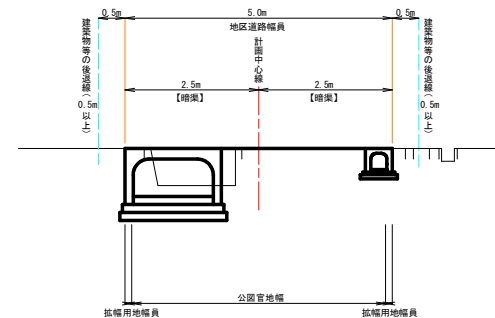
標準断面図
