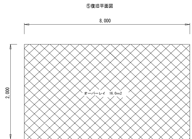
⑤アスファルト舗装復旧標準図 (t=30) アスファルト舗装 1か所 (16.0m 2 )
