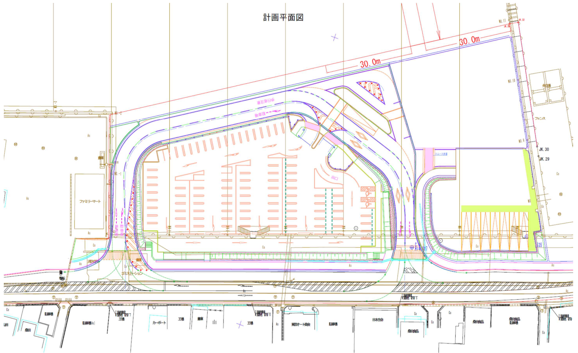
【参考2】 東側拠点 計画平面図
