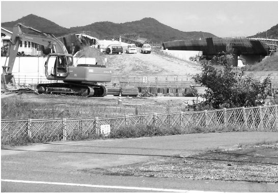
一般国道2号笠岡バイパスの工事の様子
