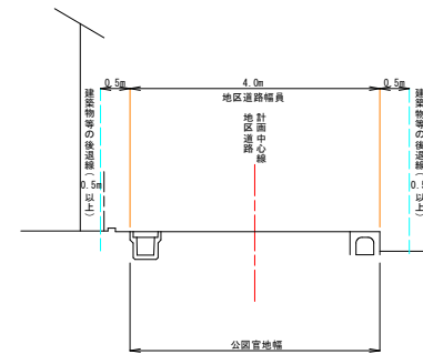
標準断面図
