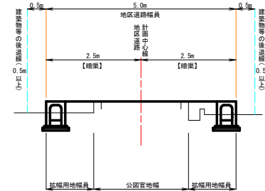
標準断面図
