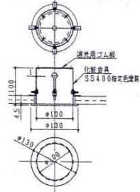
ワイヤー貫通スリーブ詳細図 (S=1/5) 規格品 DN-10 5分組 (製作)
