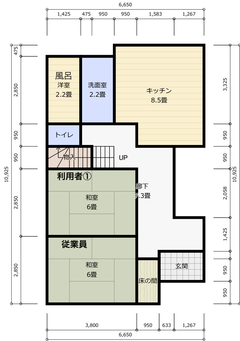
1階 縮尺 1/100
