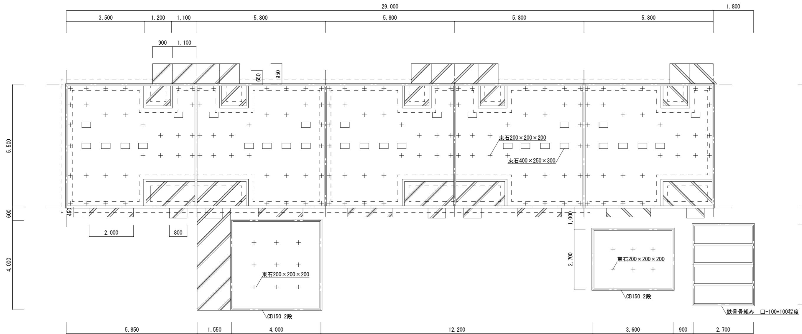
3号棟 基礎伏図 S=1/100
