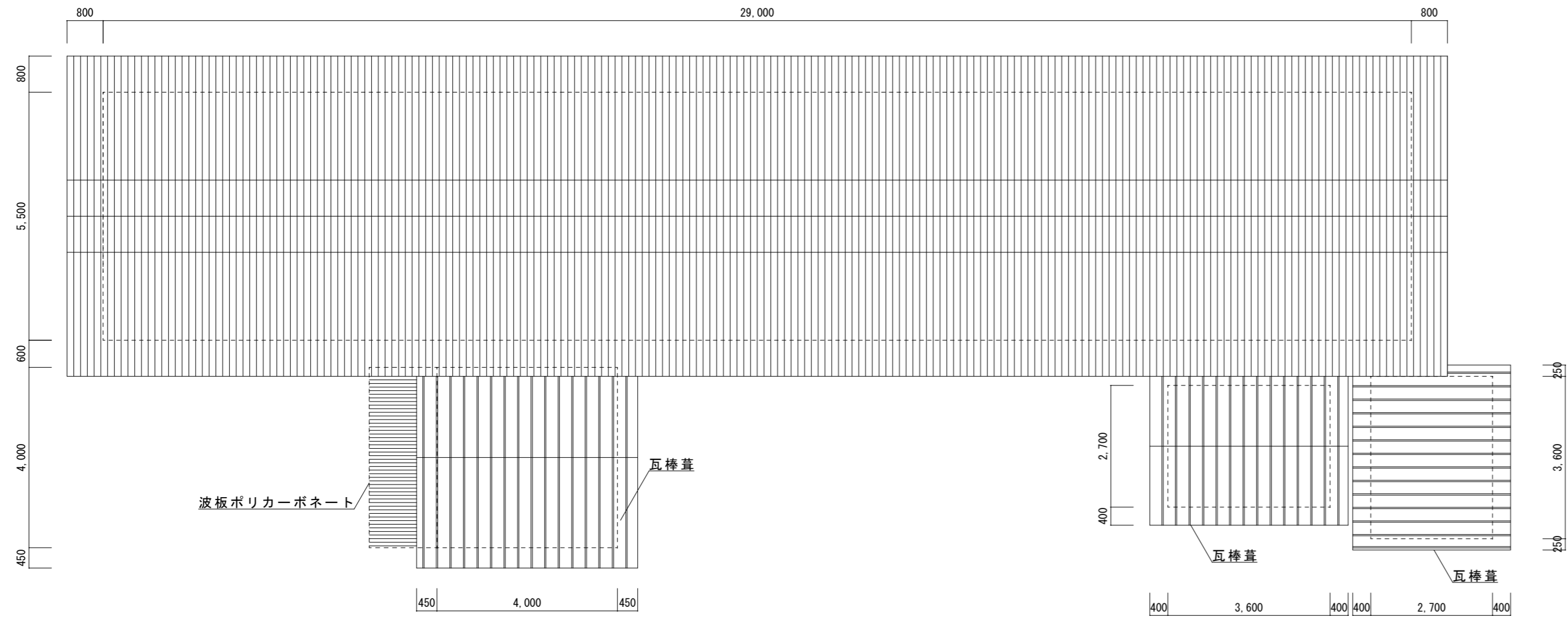
3号棟 屋根伏図 S=1/100
