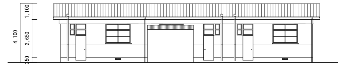
1号棟 北立面図 S=1/150
