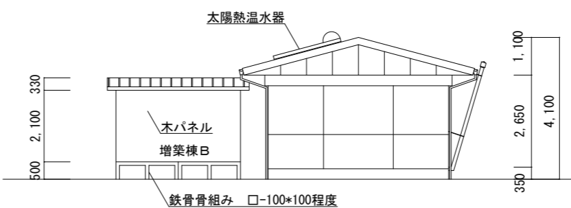
3号棟 東立面図 S=1/150
