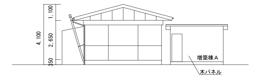
1号棟 西立面図 S=1/150
