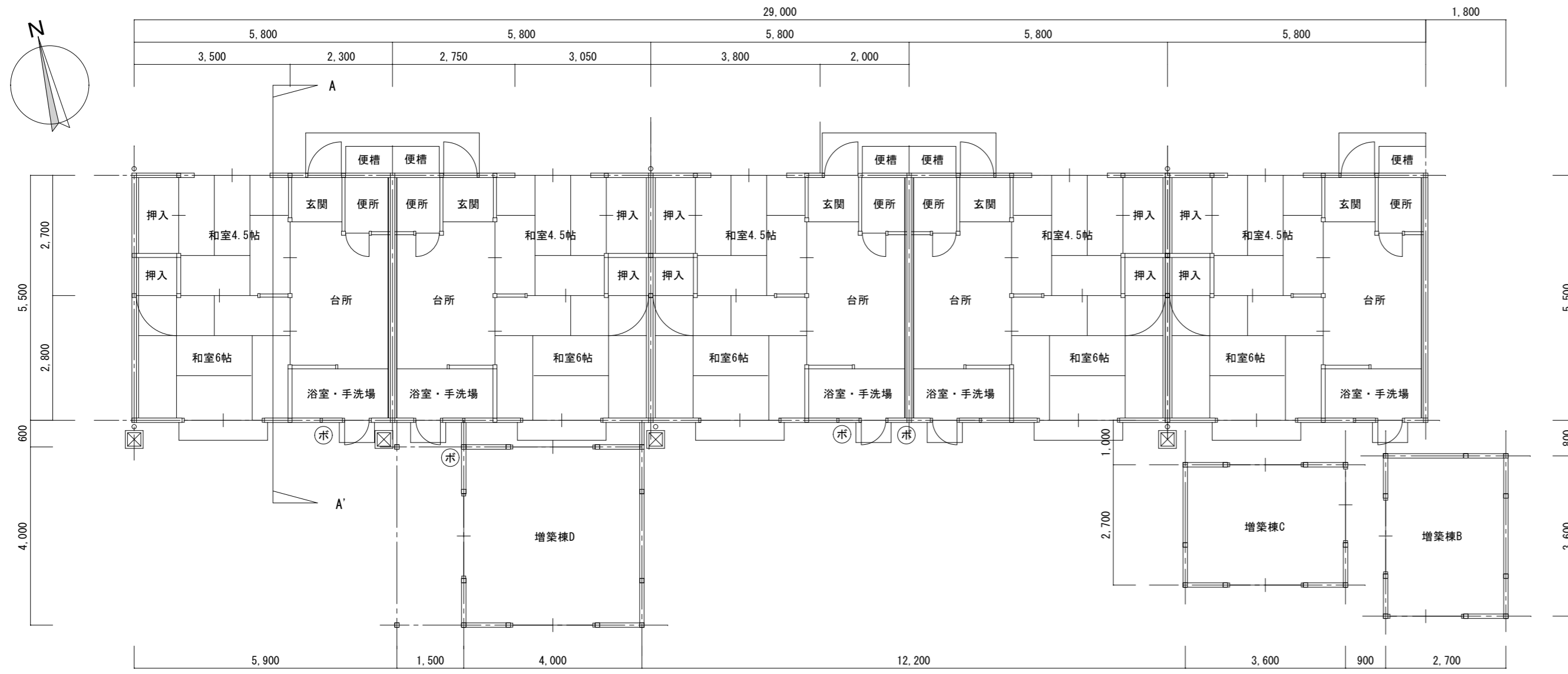
3号棟 平面図 S=1/100
