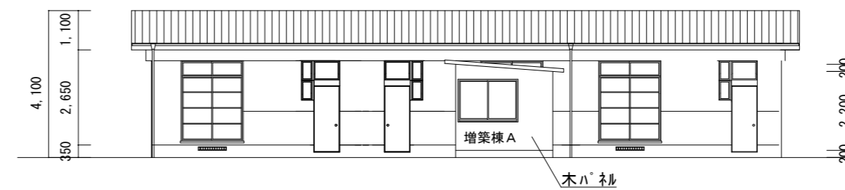
1号棟 南立面図 S=1/150
