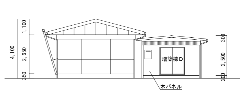
3号棟 西立面図 S=1/150
