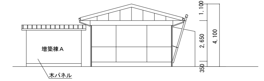
1号棟 東立面図 S=1/150
