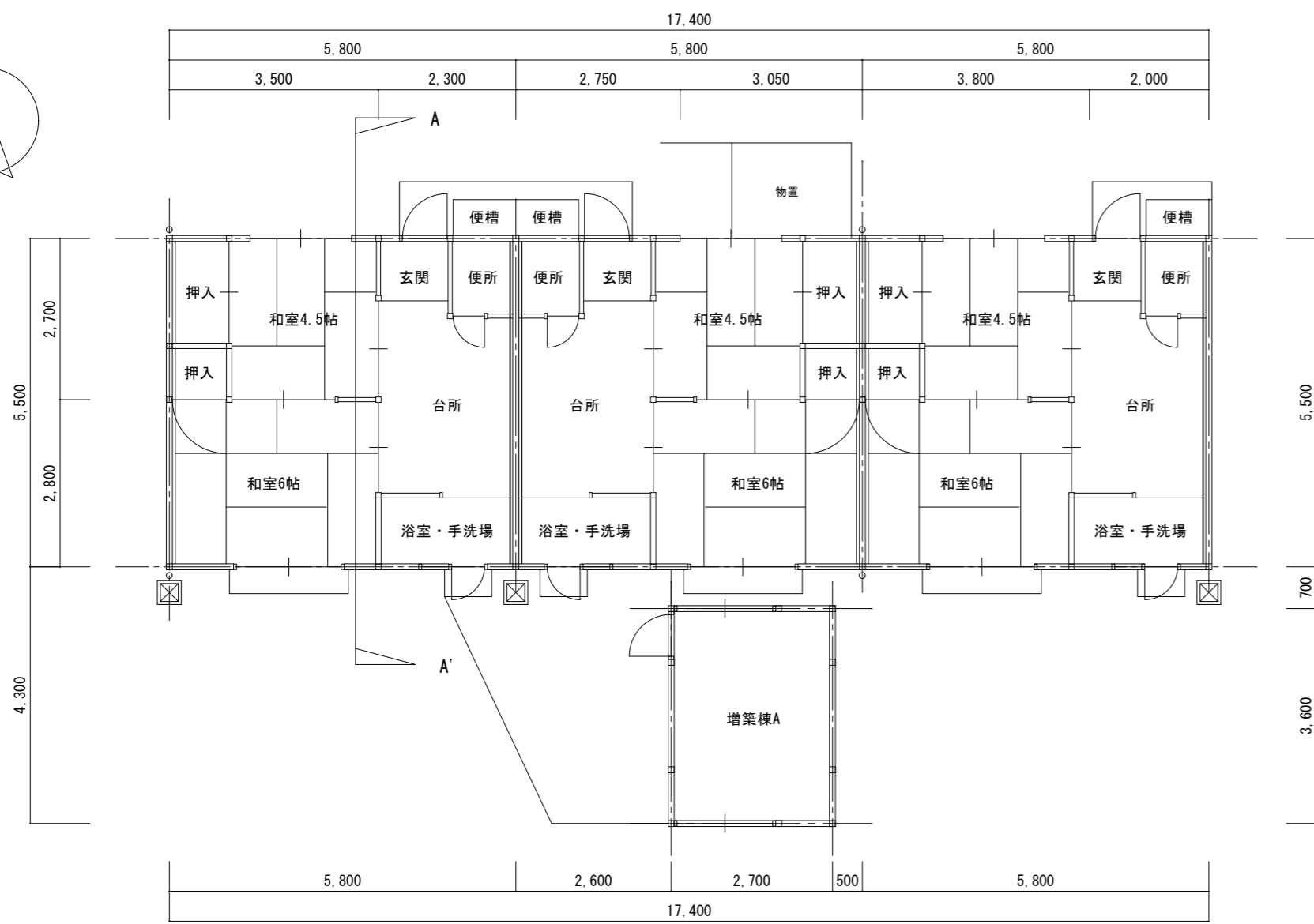
1号棟 平面図 S=1/100
