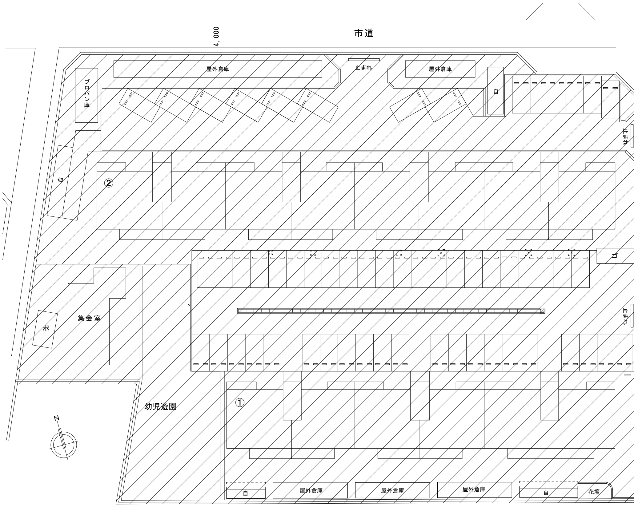
配置図 S=1/300
