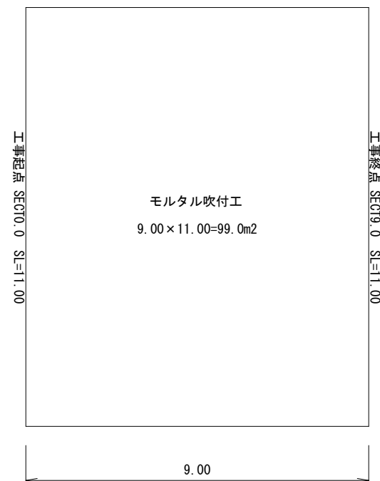
展開図(モルタル吹付) S=1:100
