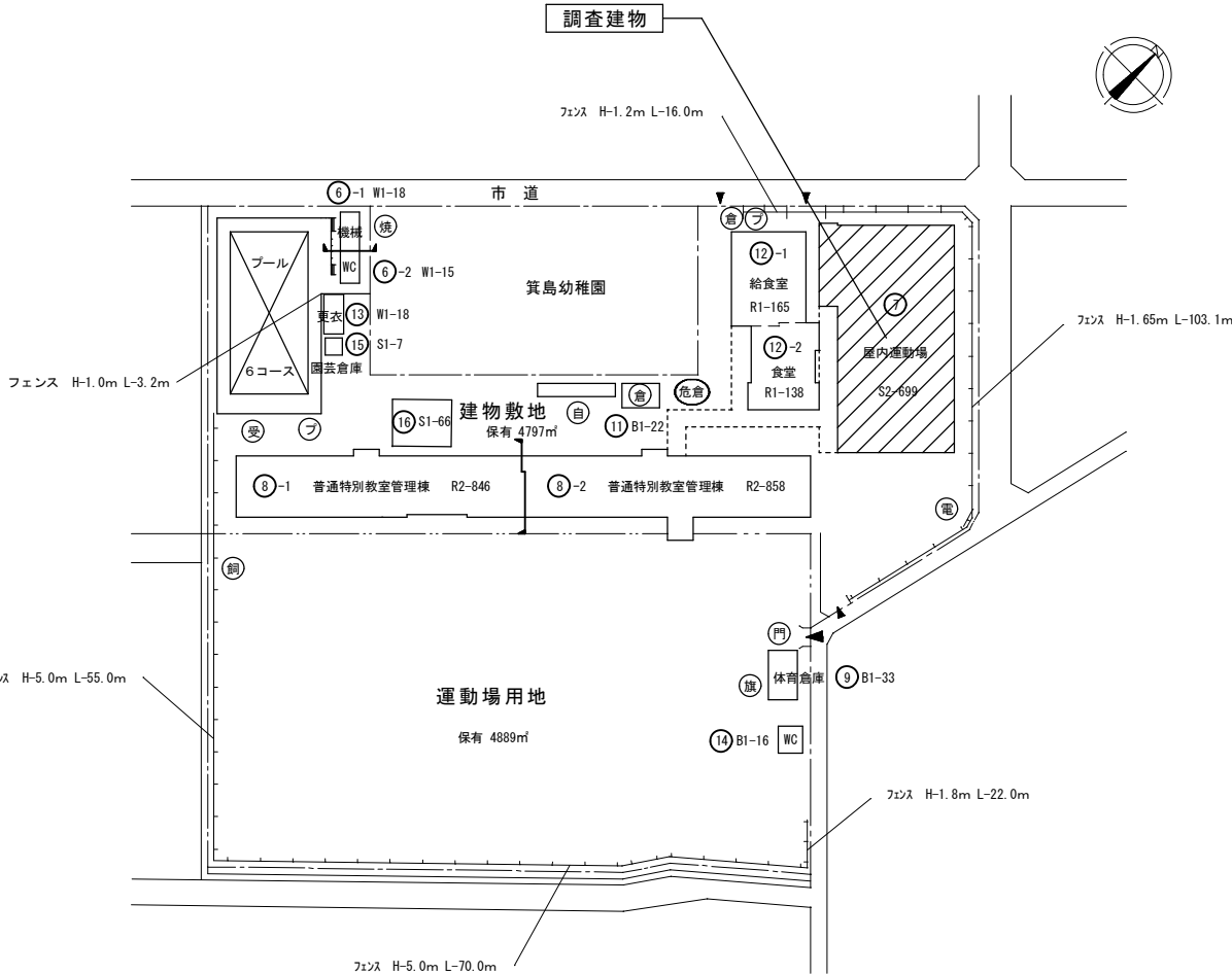
配置図 S=1/600
