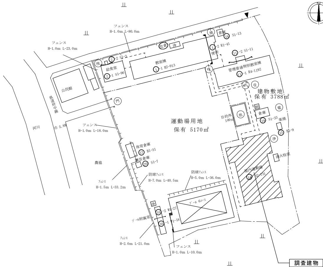
配置図 S=1/600
