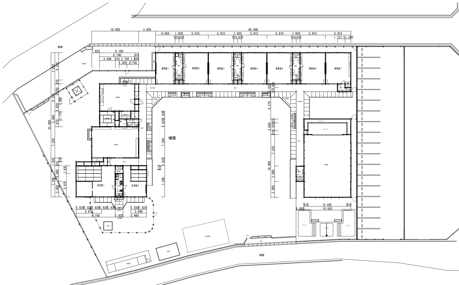
配置平面図 1:300
