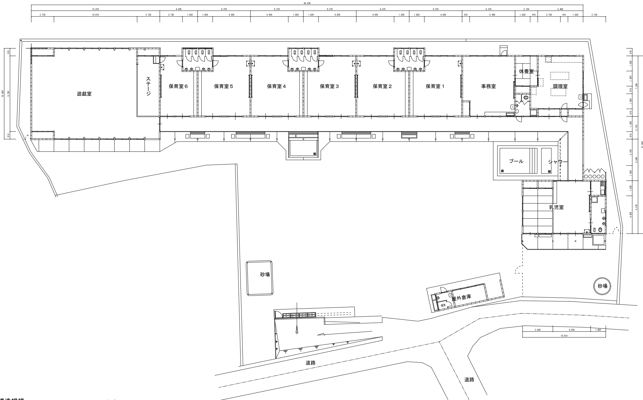
配置平面図 1:200
