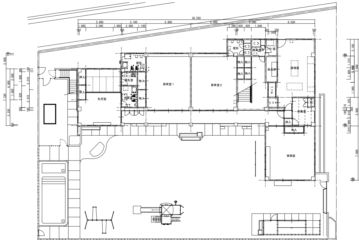
1階配置平面図 1:200
