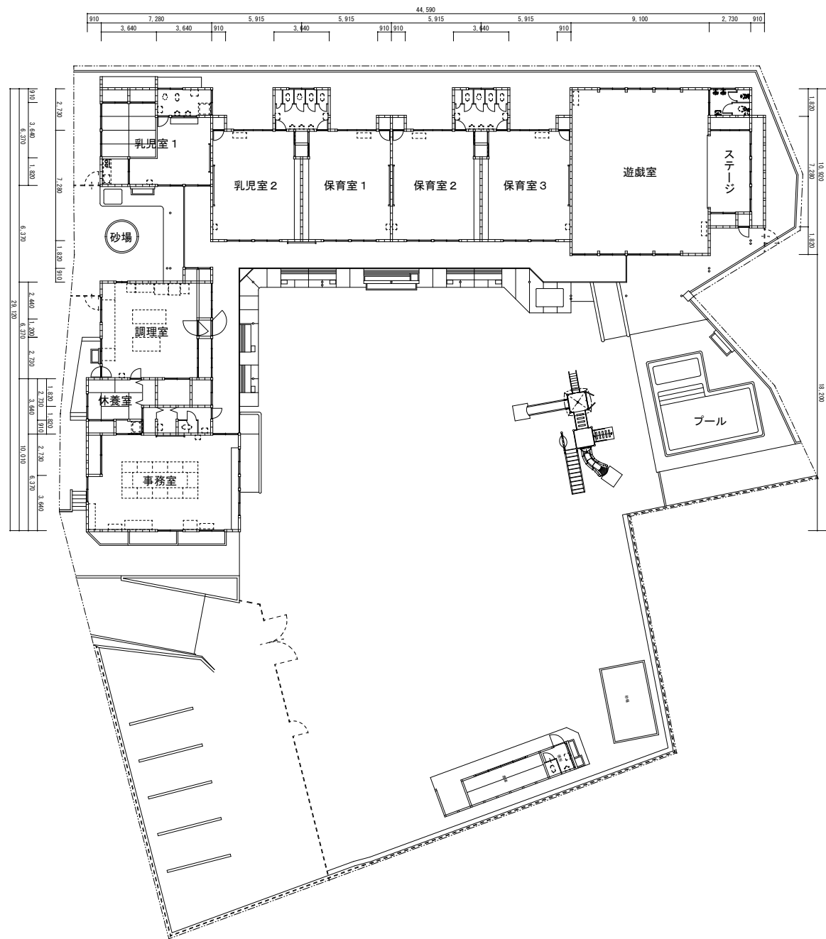
配置平面図 1:200
