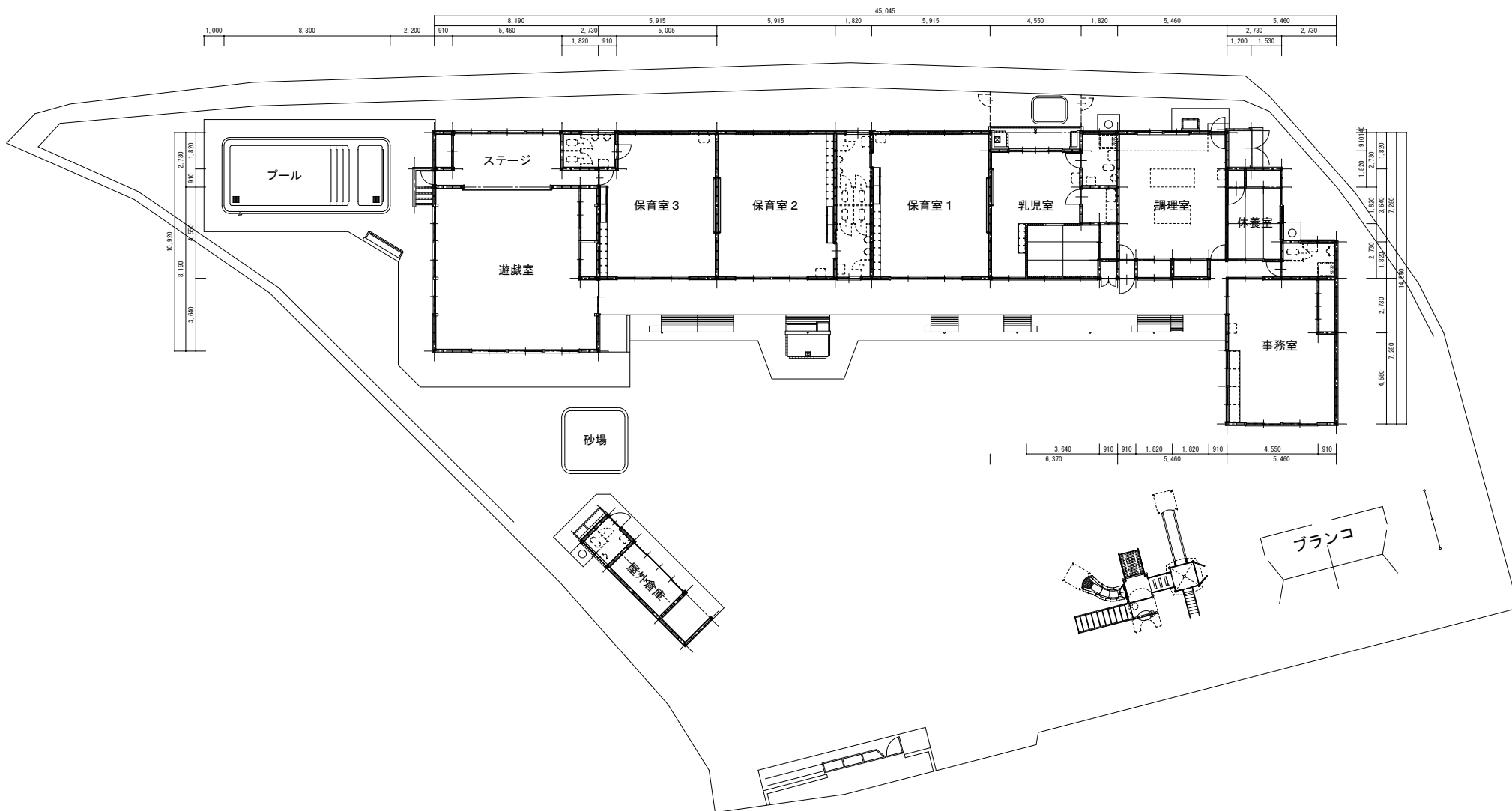
配置平面図 1:200
