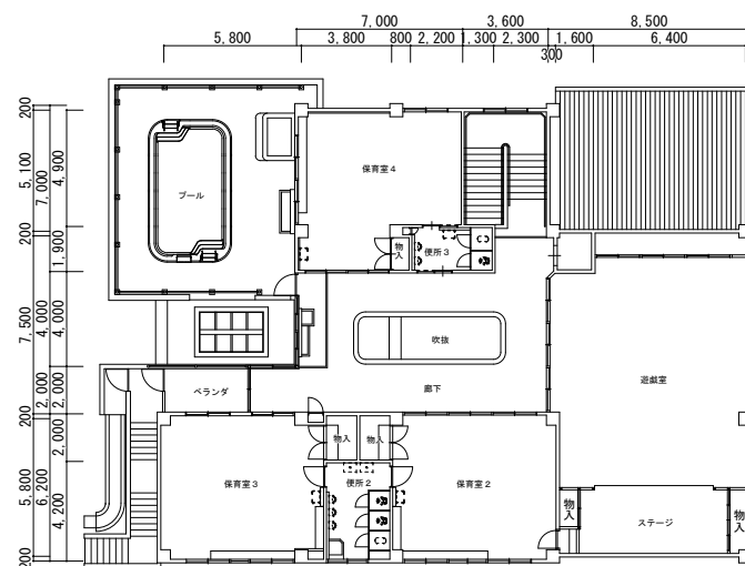
2階平面図 1:250
