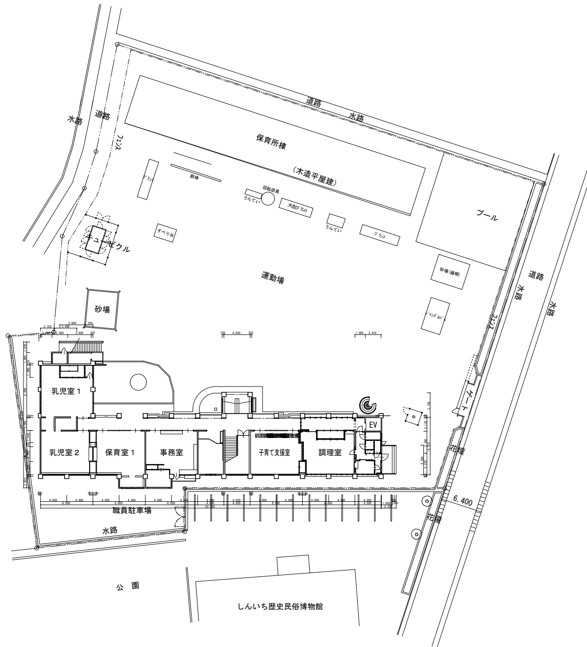
1 階配置平面図 1:400
