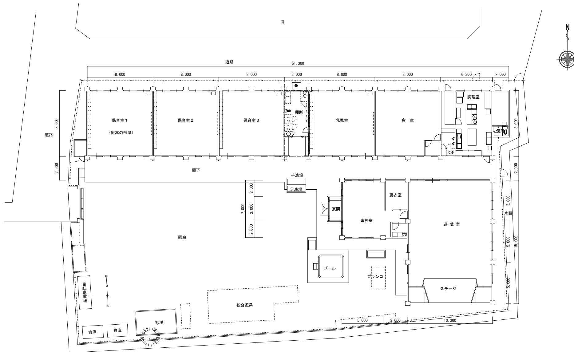
配置平面図
