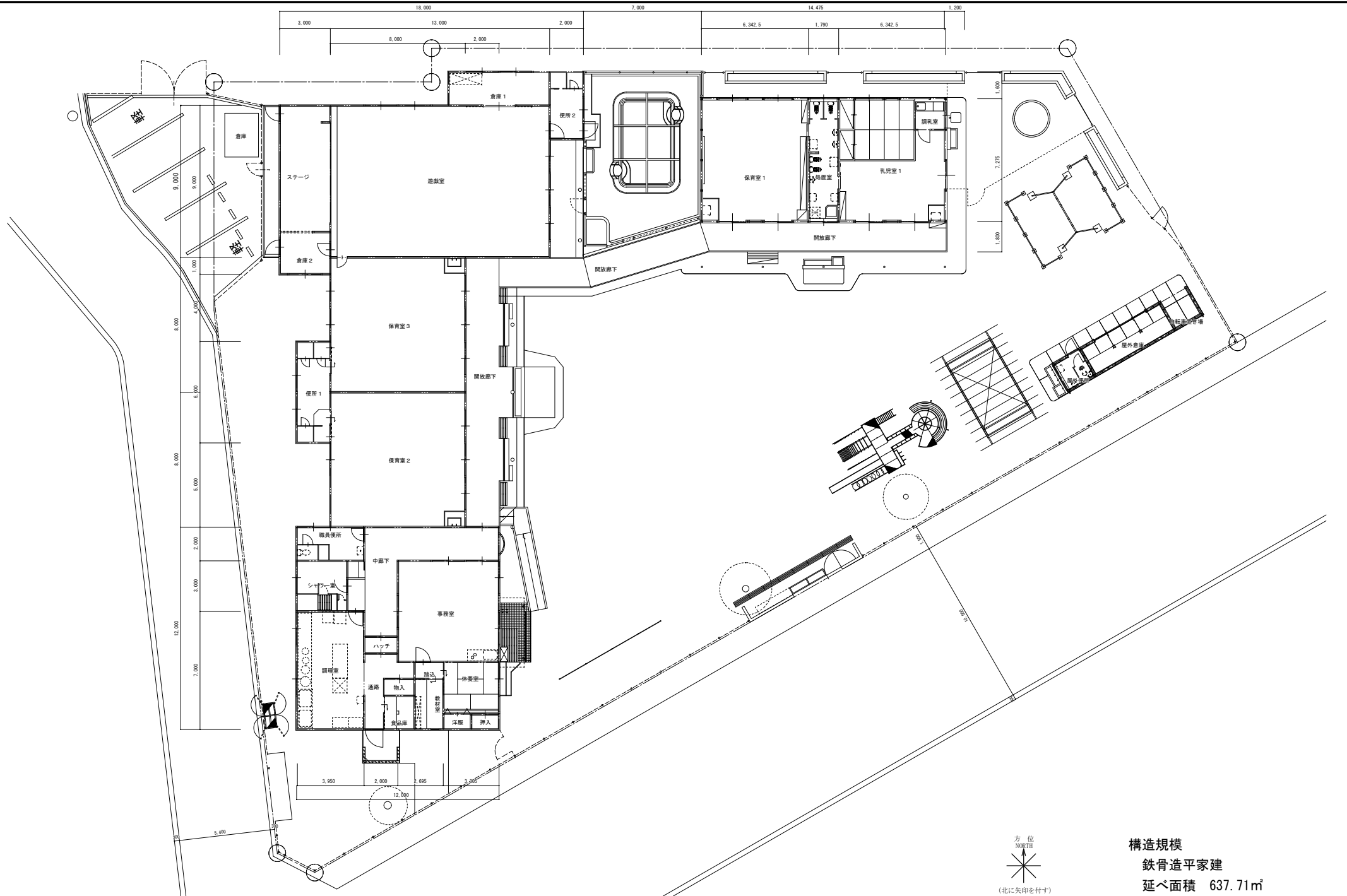
配置平面図 1:200
