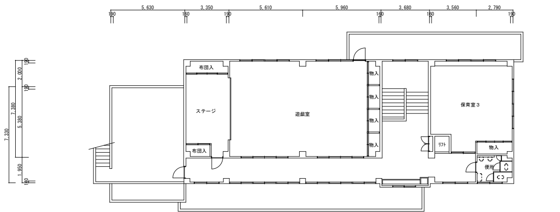
2階平面図 1:200
