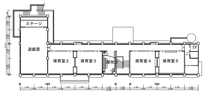
2 階平面図 1:400
