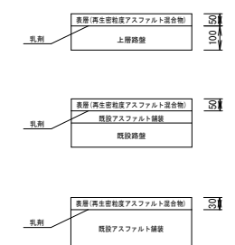
舗装標準断面図 S=1:20
