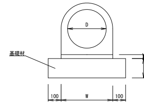
台付鉄筋コンクリート管 D300 S=1:20
