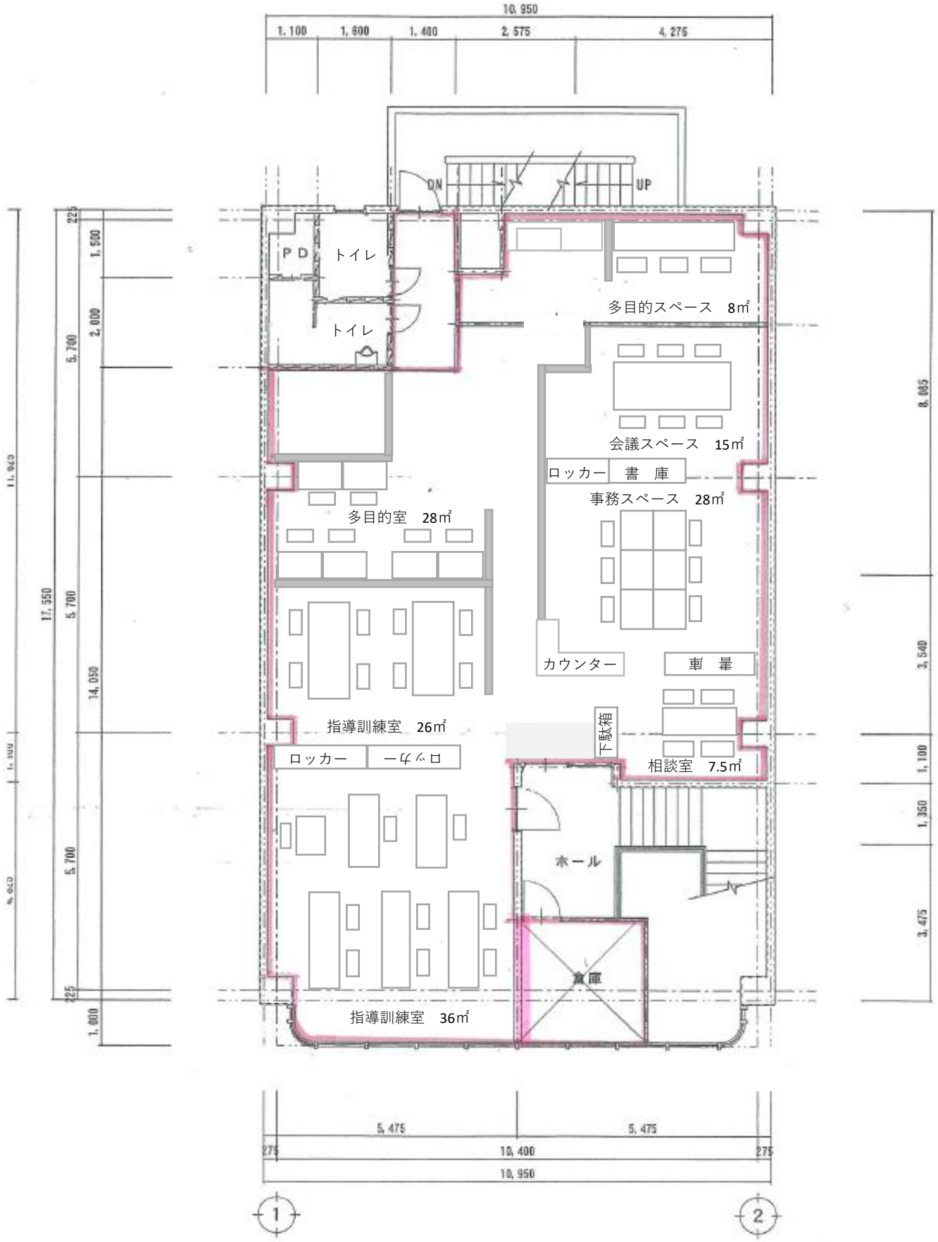
4階 平面図 1:100
