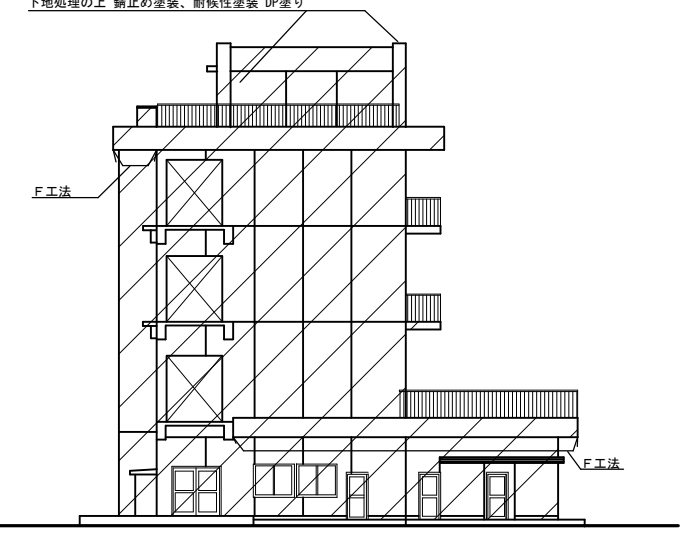
西立面図 1/150
