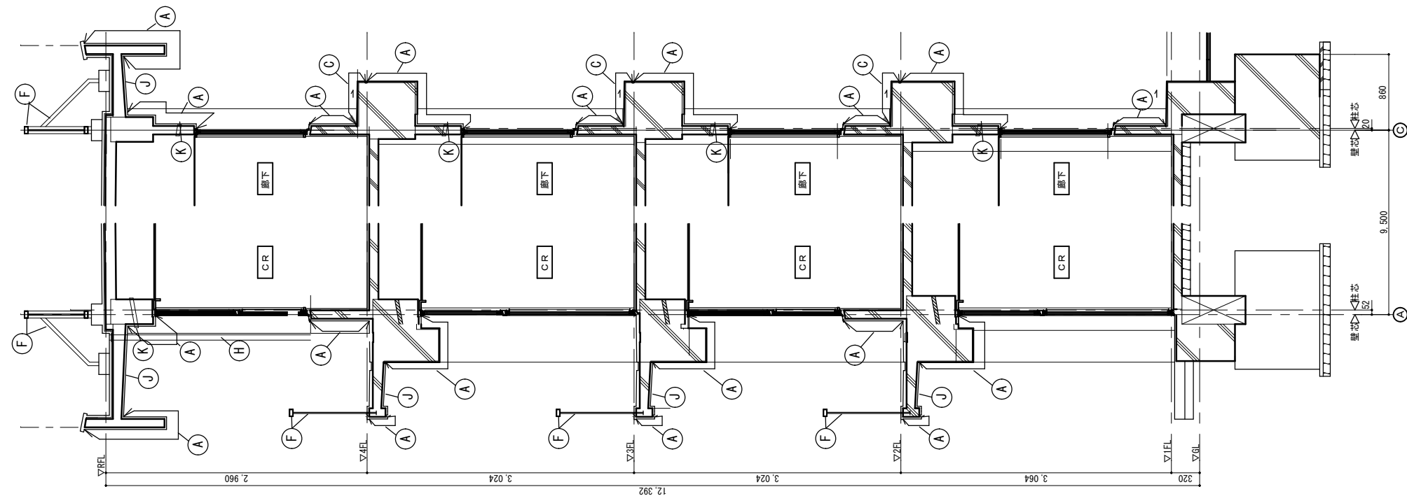
X6~X10 矩計図 S=1/30 (新置フレーム部)
