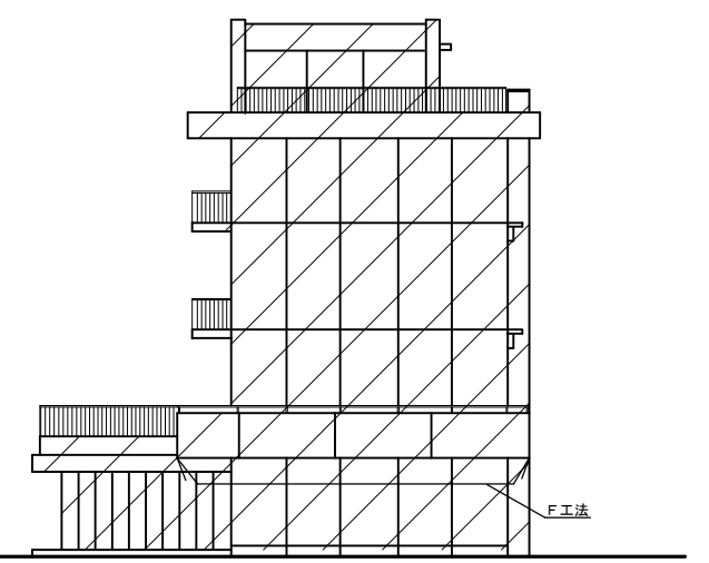
東立面図 1/150
