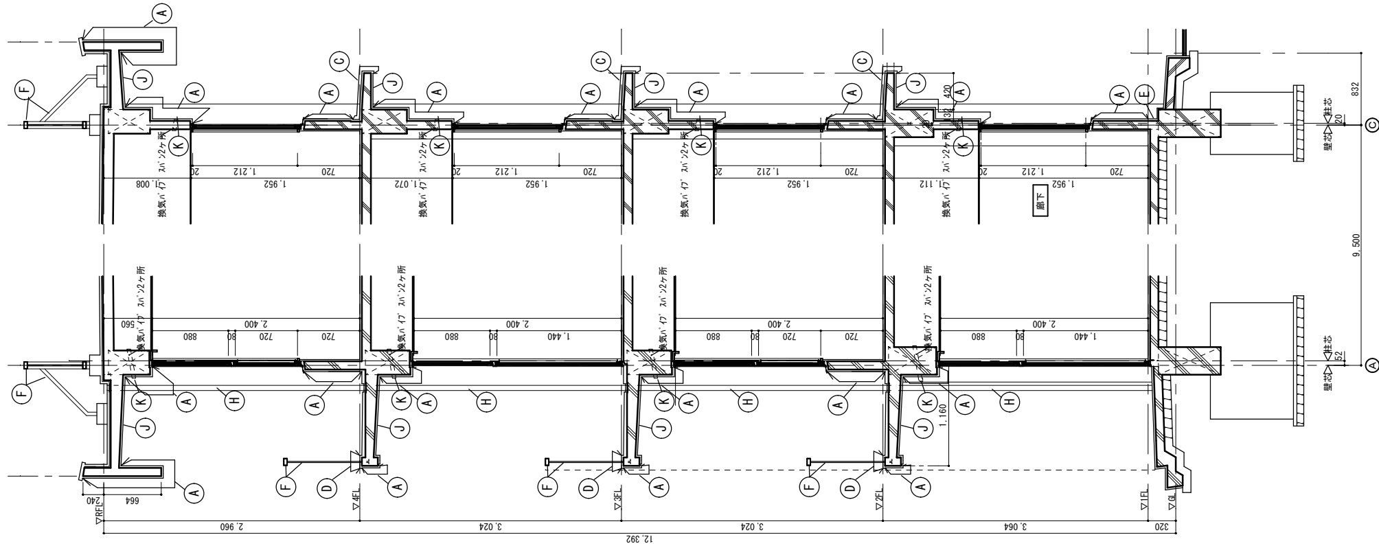
X6~X10 矩計図 S=1/30 (一般部)
