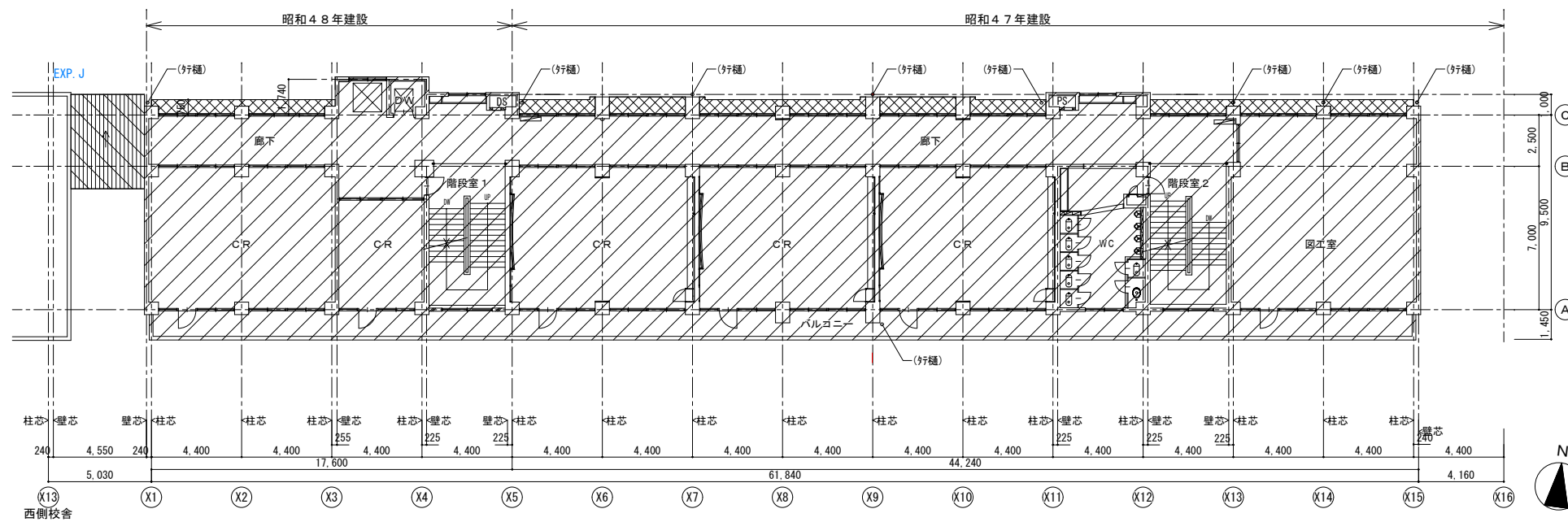
4階平面図 1/150
