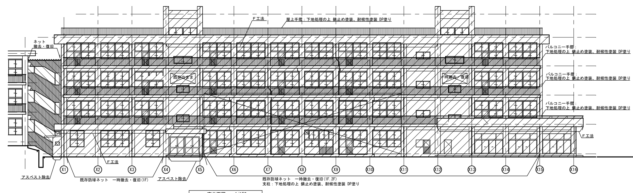
南立面図 1/150
