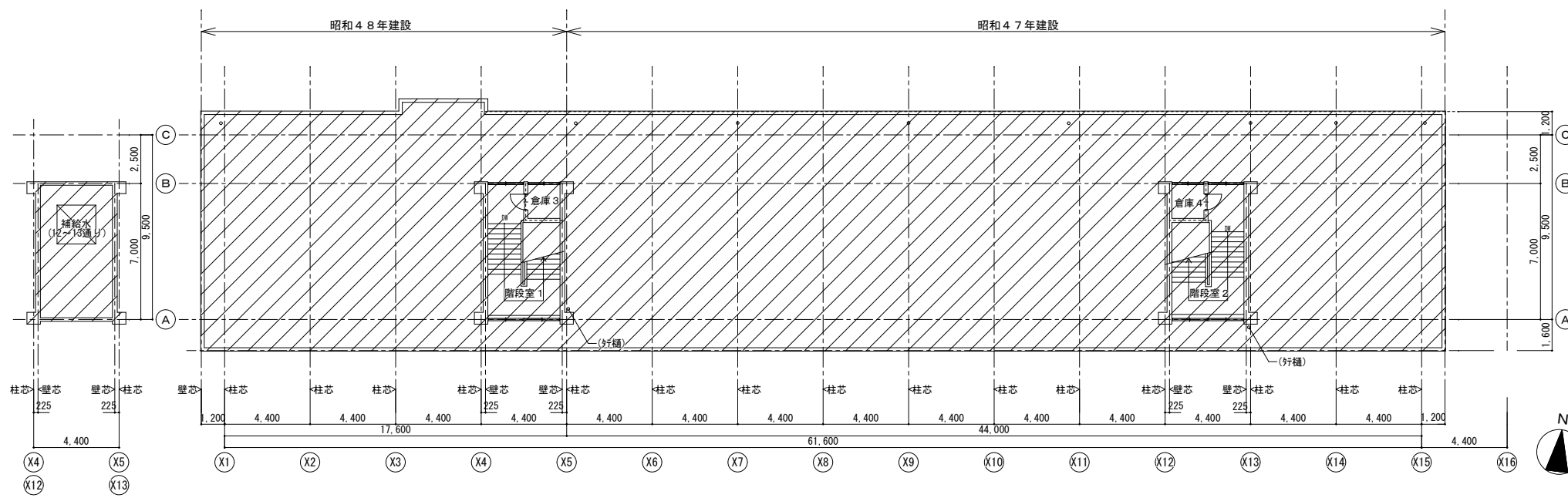
R階平面図 1/150
