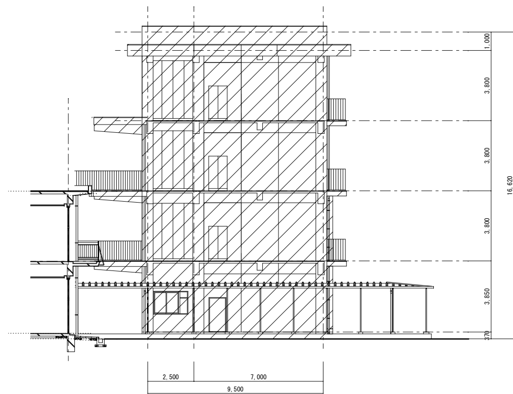
西立面図 1/100
