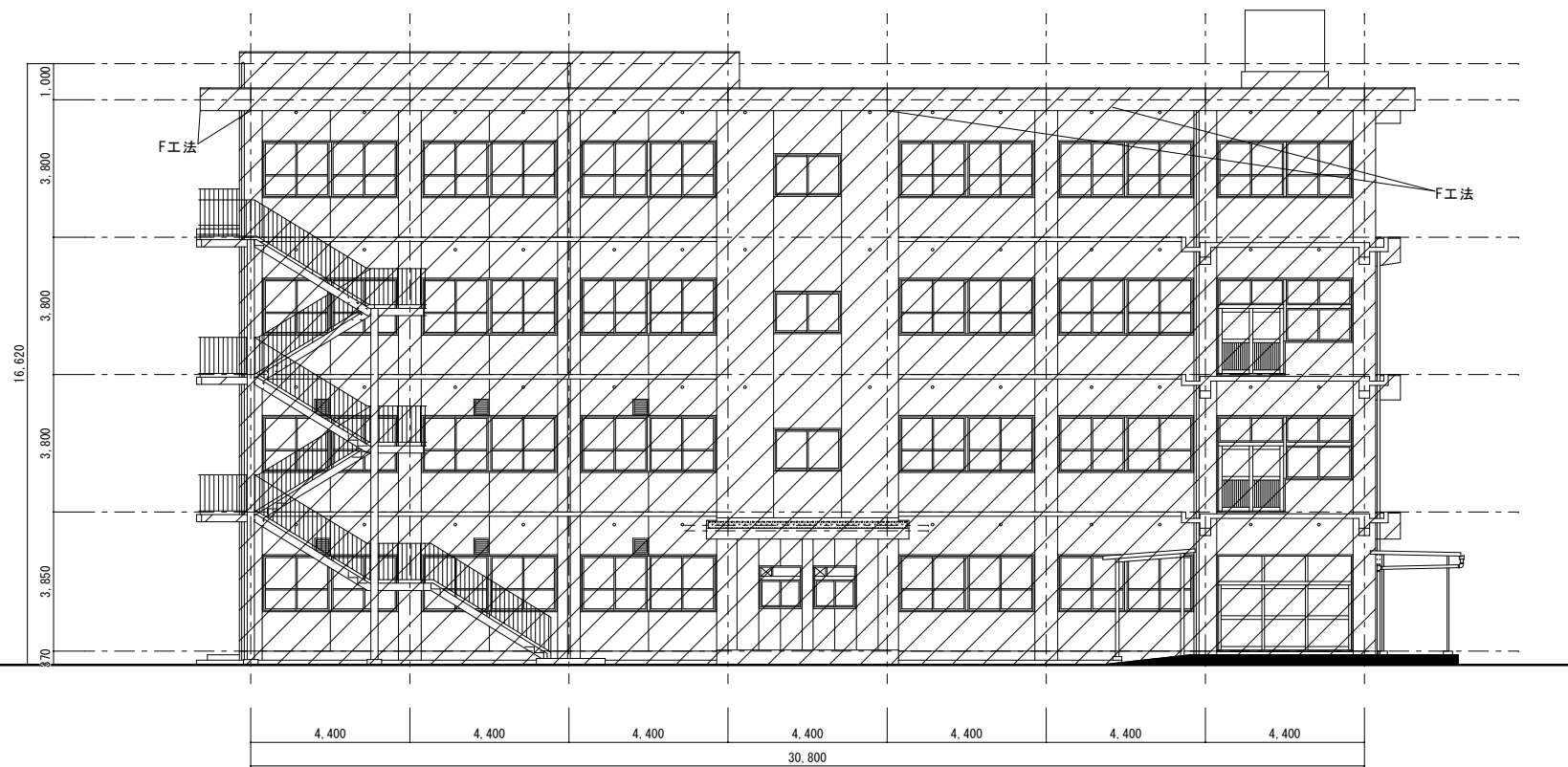
北立面図 1/100
