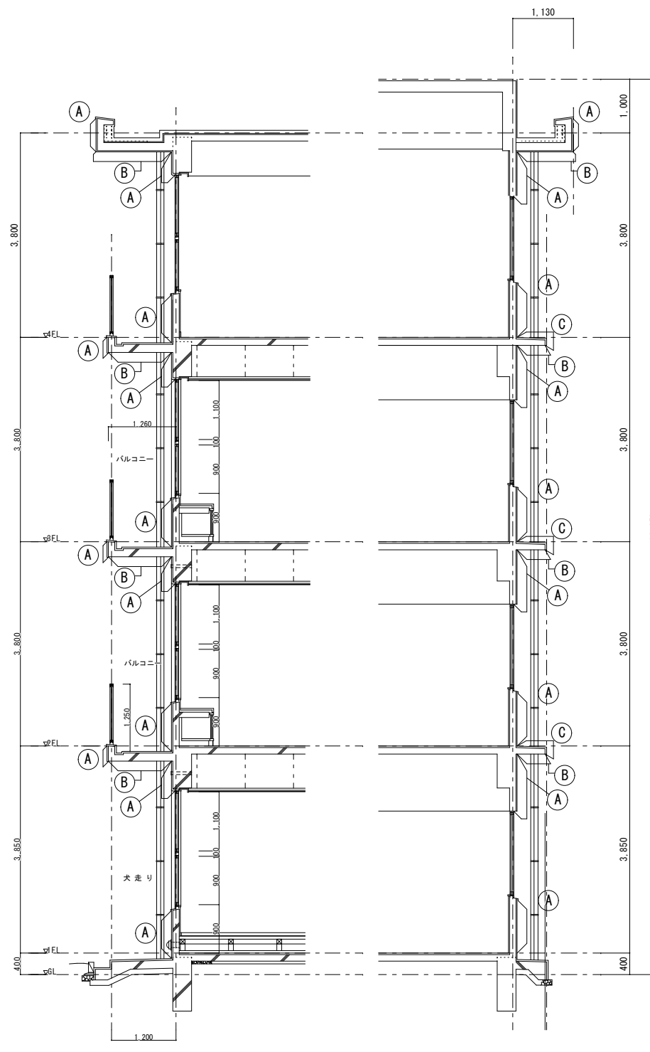
断面詳細図 S=1:50
