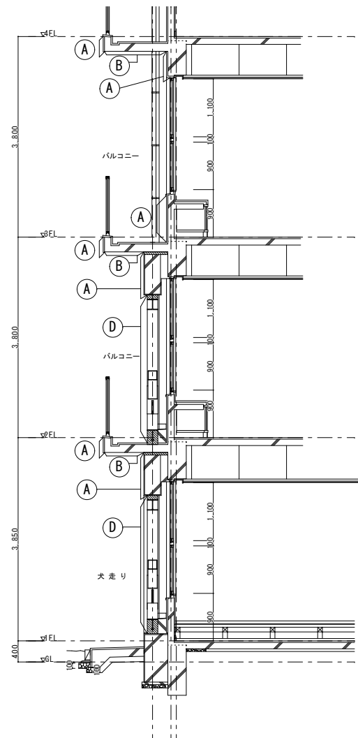
断面詳細図 S=1:50
