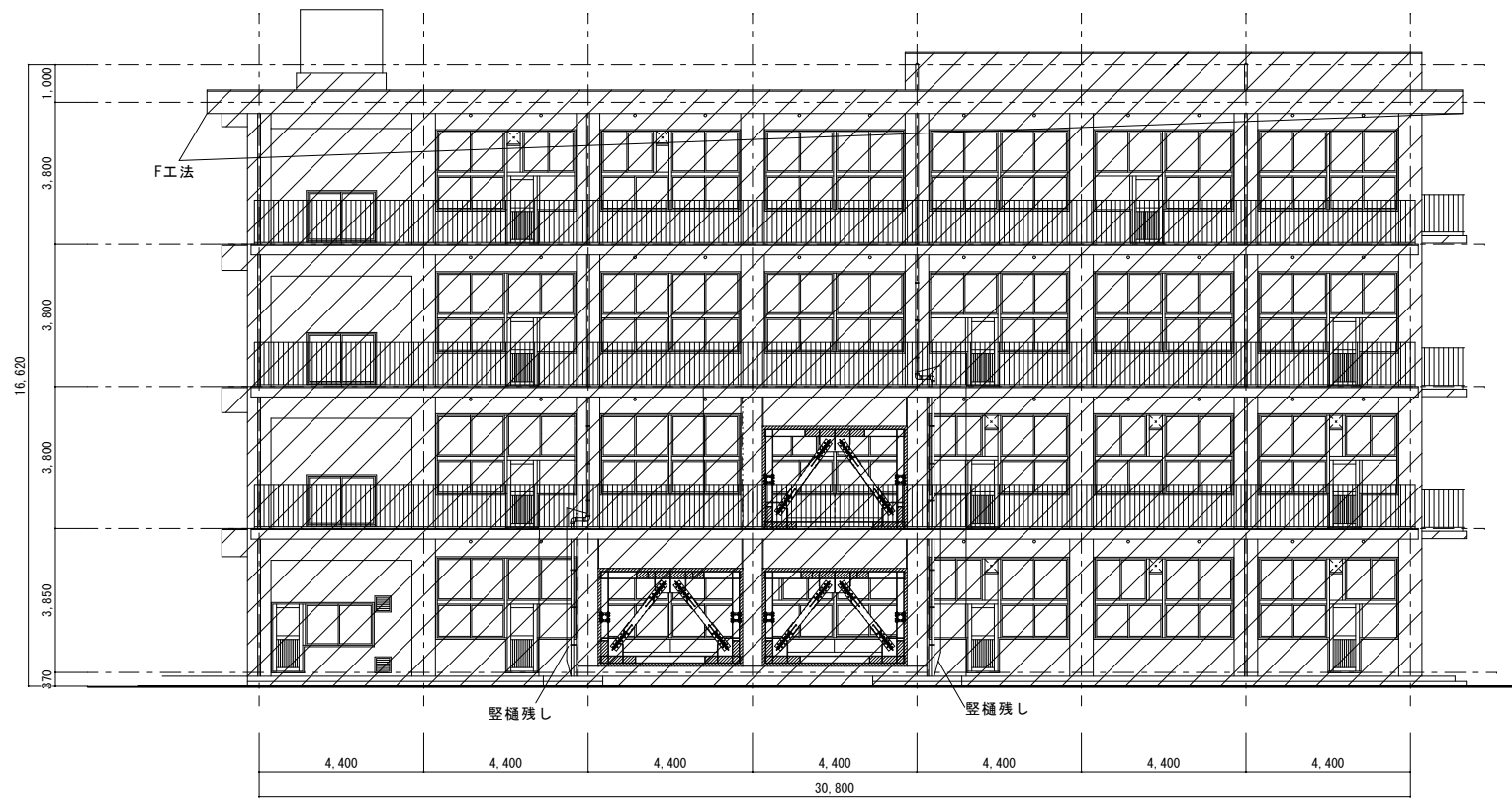
南立面図 1/100
