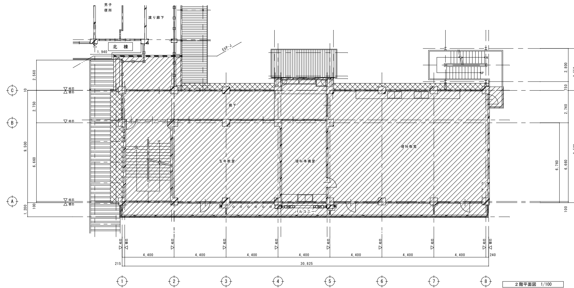
2階平面図 1/100
