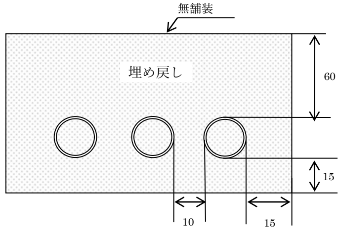
図2 埋設構造例
