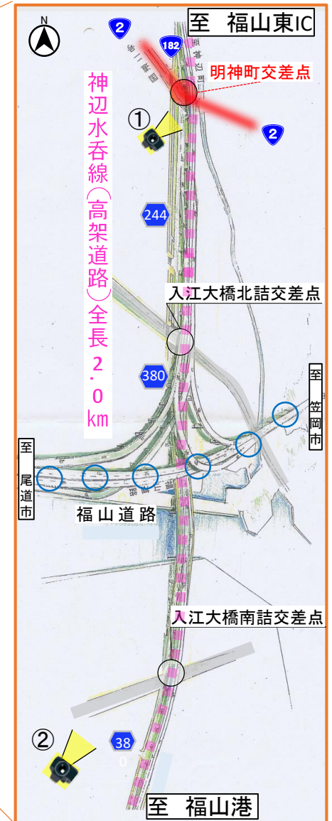
神辺水呑線計画図
