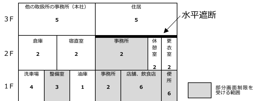
建築物の面積制限の例図 (注 太字の数字は適用される号の例)
