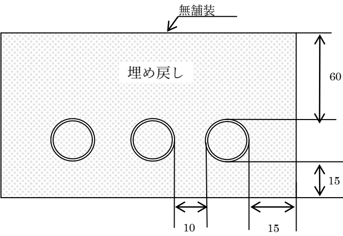
図 2 埋設構造例
