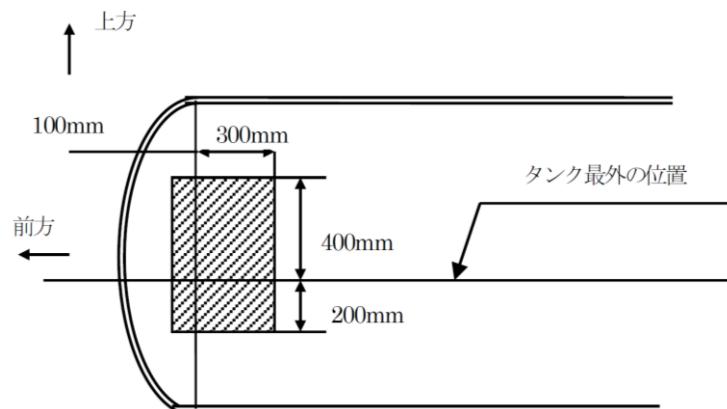
図第3-6-9 タンク本体の応力集中防止範囲
