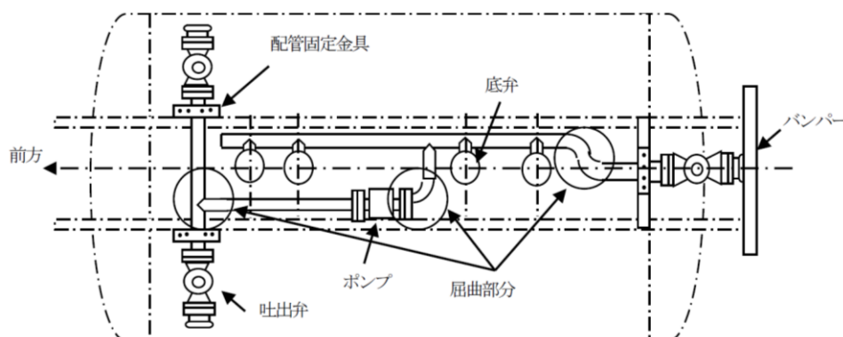
図第 3-6-40 配管による底弁に直接衝撃が加わらない措置
