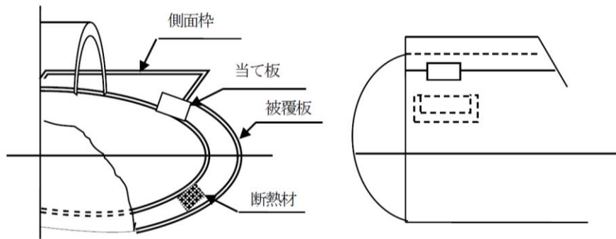
図第 3-6-22 タンク胴板に直接取り付ける側面枠の方法
