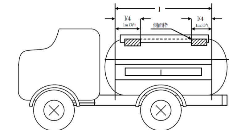
図第 3-6-18 単一車形式の移動タンク貯蔵所の側面枠の取付位置
