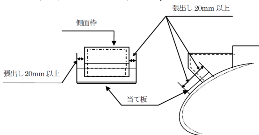
図第 3-6-16 箱形の側面棹に設ける当て板の取付方法
