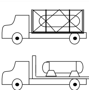
図第3-6-3 単一車形式で積載式の移動タンク貯蔵所の例
