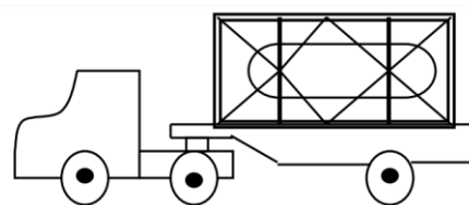
図第3-6-4 被けん引車形式で積載式の移動タンク貯蔵所の例
