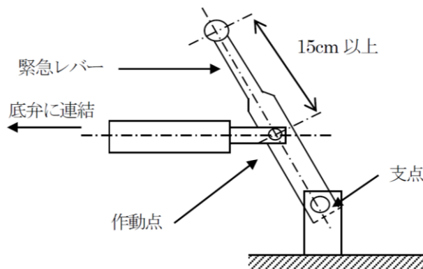
図第 3-6-34 緊急レバーの構造
