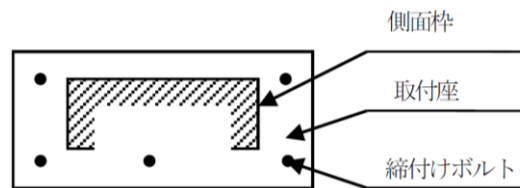
図第 3-6-26 1 の締付けボルトに応力集中が発生しない締付け配列方法
