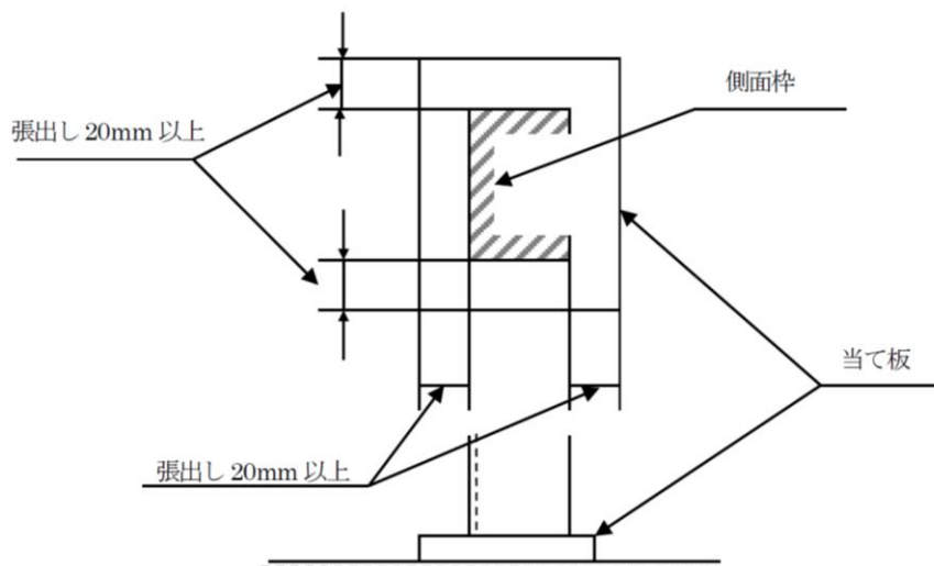
図第 3-6-17 棒形の側面枠に設ける当て板の取付方法
