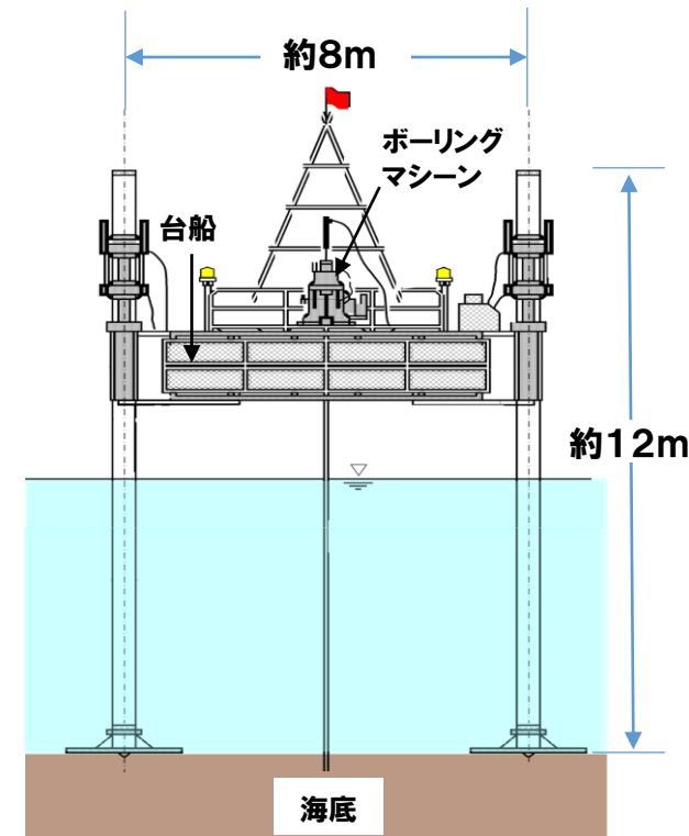
土質調査で使用する台船 ※12月6日(金)頃から掘削開始予定
