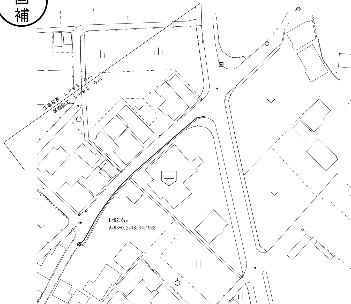
平面図 S=1:1,000
