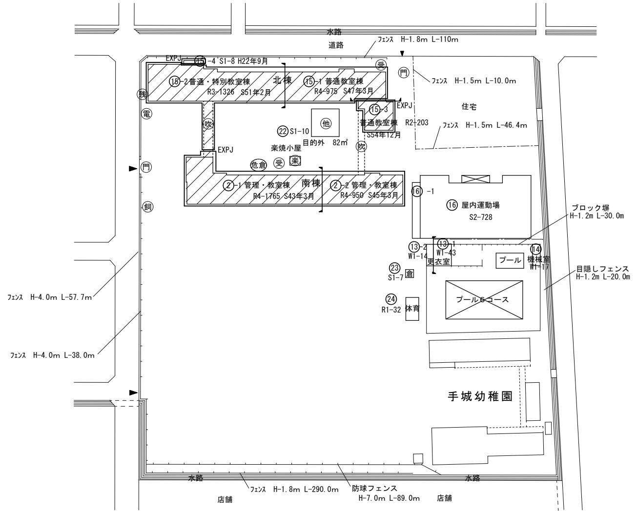
配置図 S=1/600
