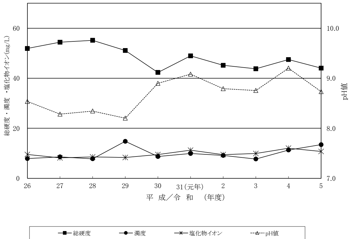
箕島浄水場 原水
