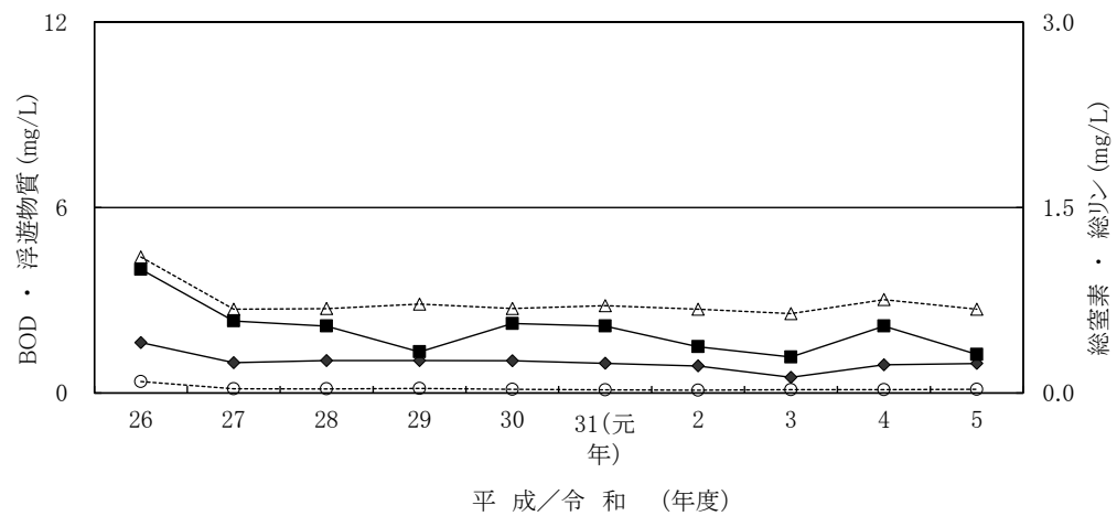
芦田川表流水 ・ 久佐地点
