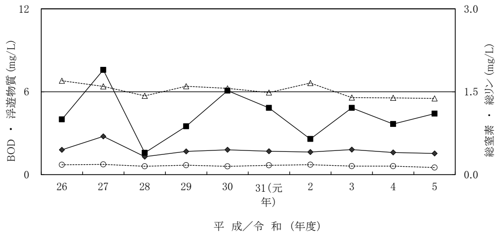
高屋川表流水 ・ 横尾地点
