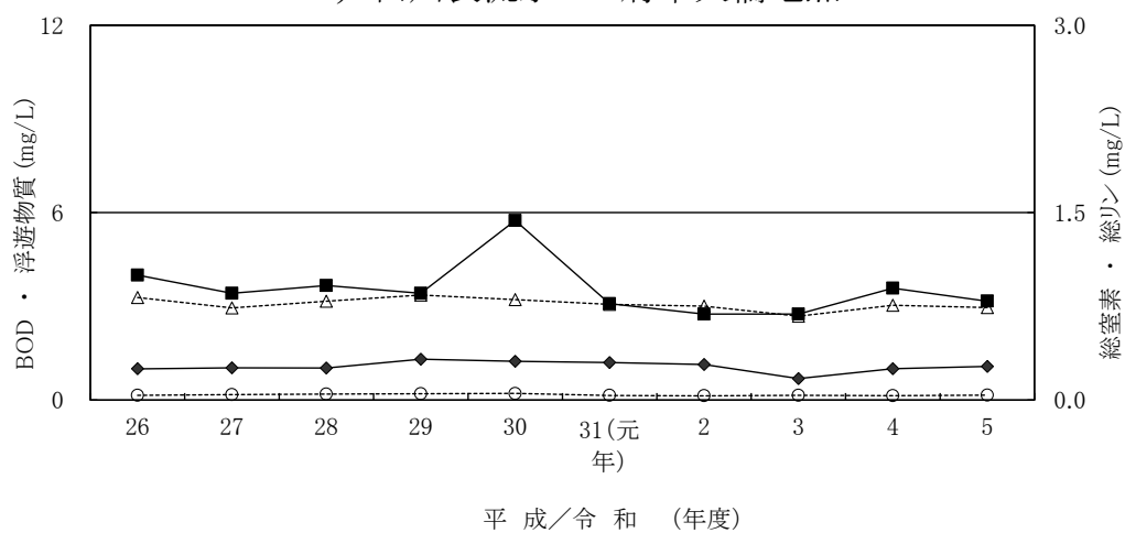
芦田川表流水 ・ 府中大橋地点
