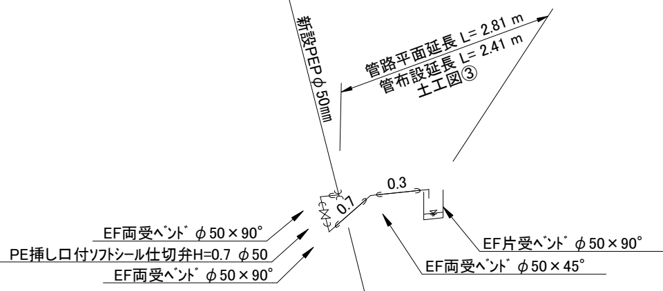
③ドレン配管図
