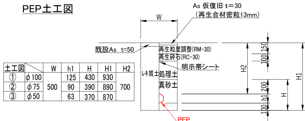
PEP土工図
