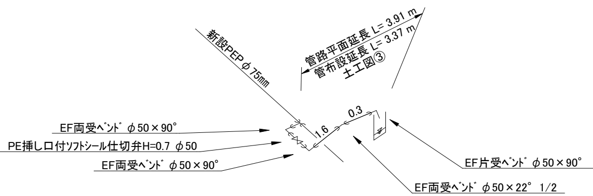
①ドレン配管図
