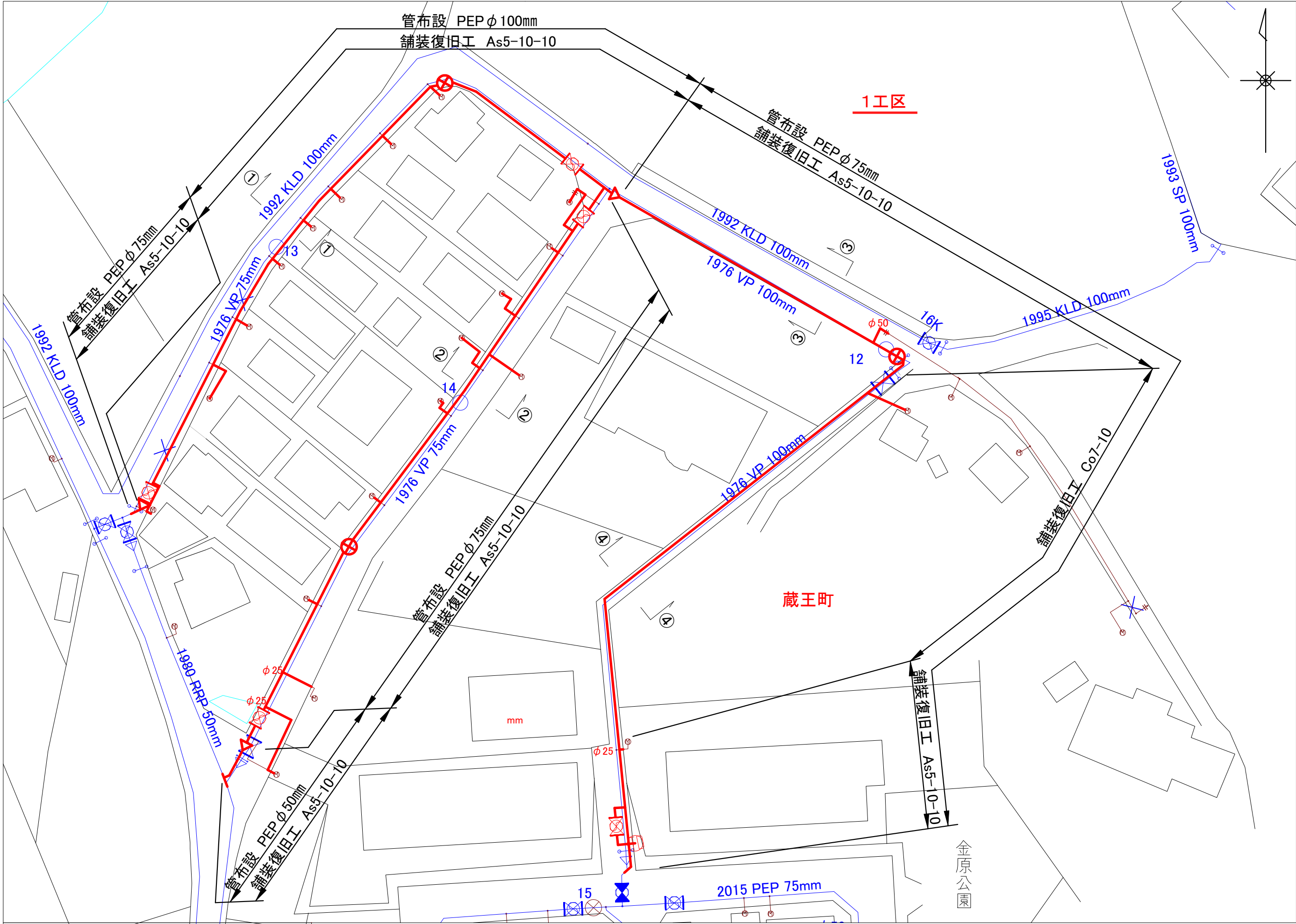
1工区・3工区平面図 S=1/600
