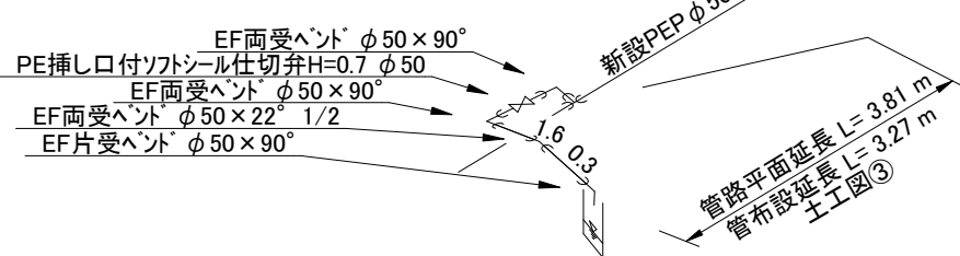
②ドレン配管図
