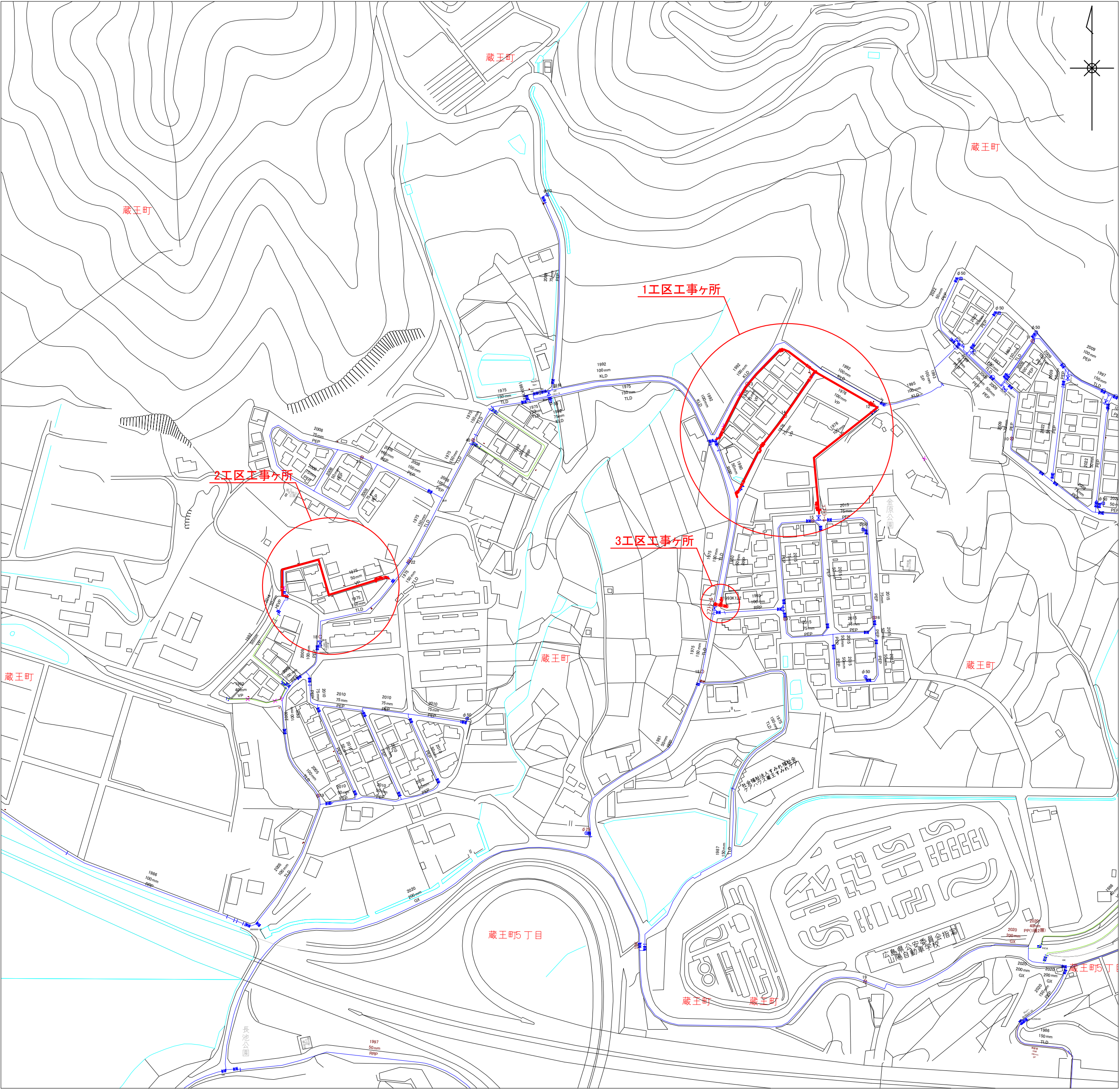
配管図 S=1/2,500
