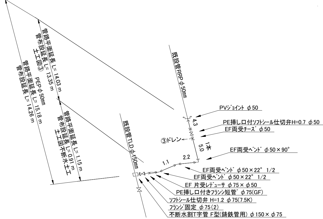
3工区配管図
