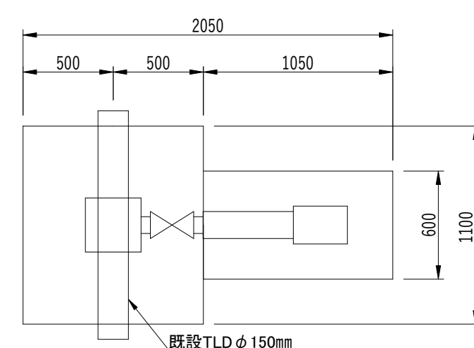
不断水土工平面図
