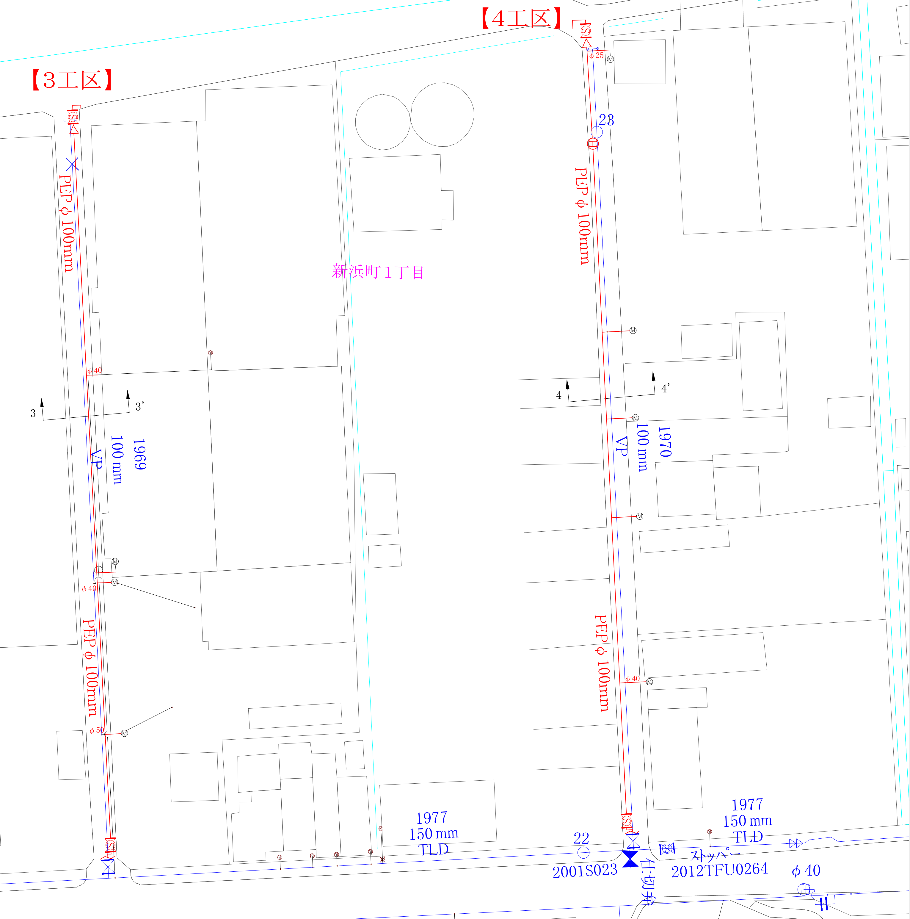
横断面図(2)
