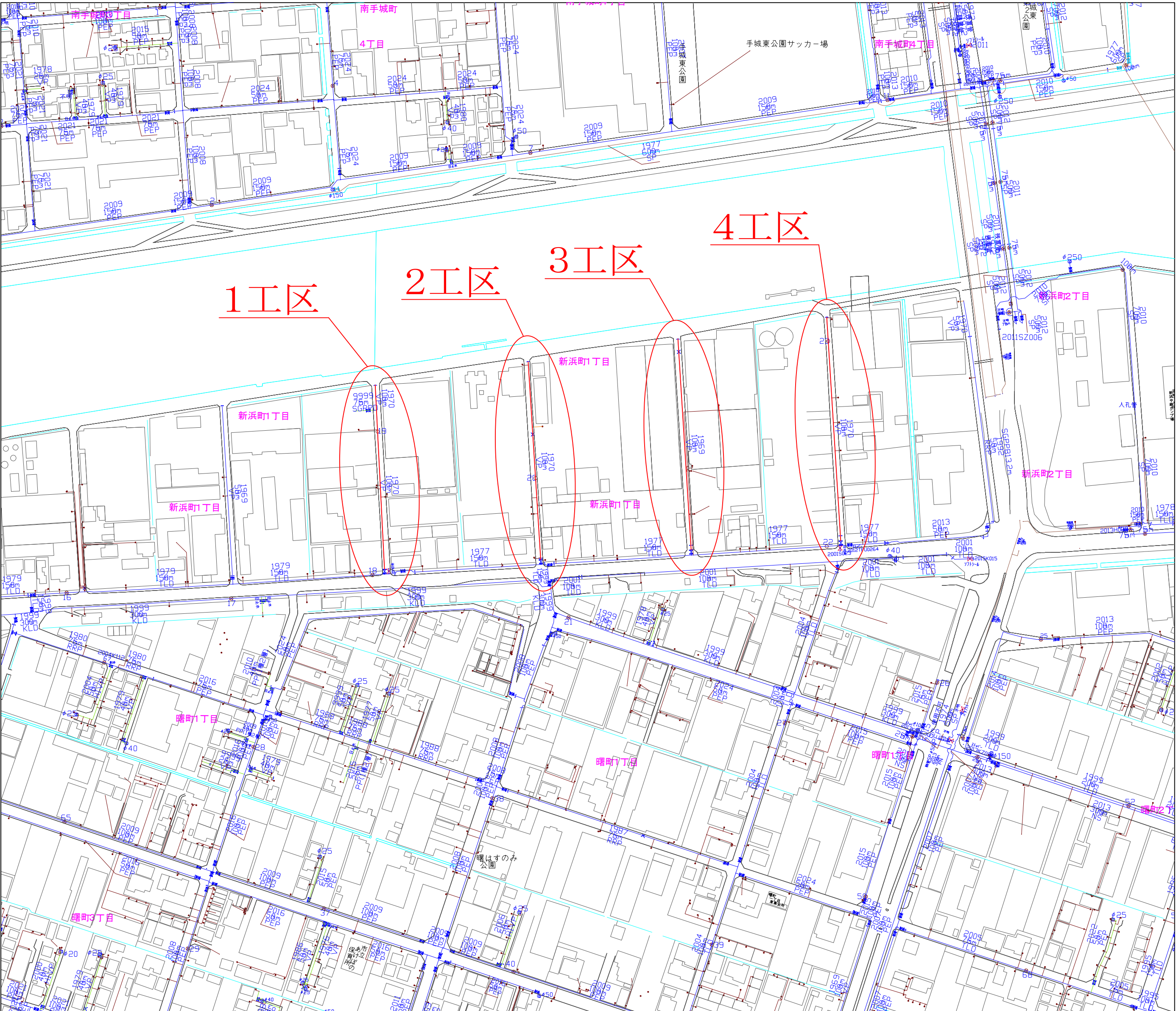
配管図 S=1/2500
