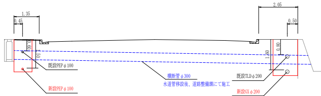
土工図 S=1/30
