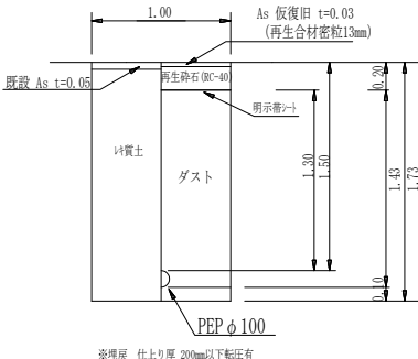
PEP φ100土工図
