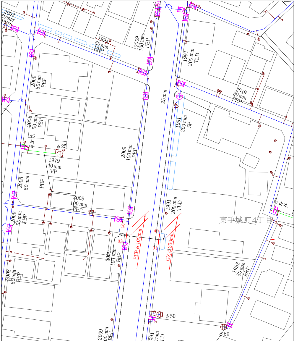
平面図 S=1/500
