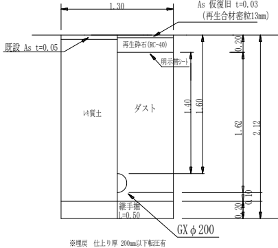
土留工 標準図 S=NON
