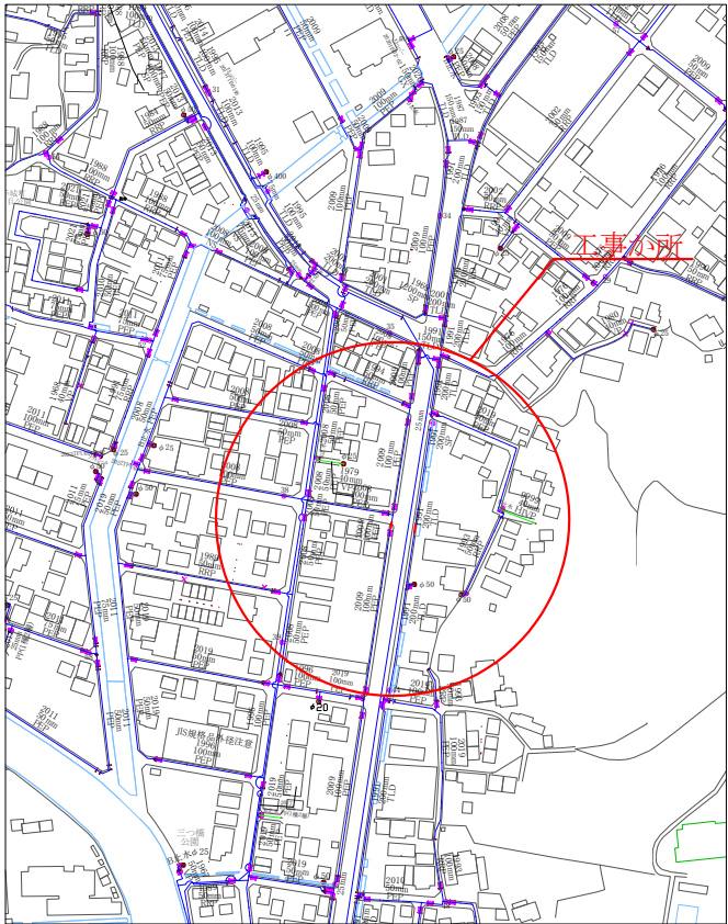
配管図 S=1/2500
