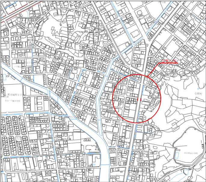
配管図 S=1/2500
