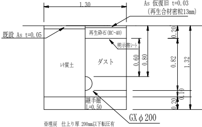
GX φ200土工図 (土工図②)
