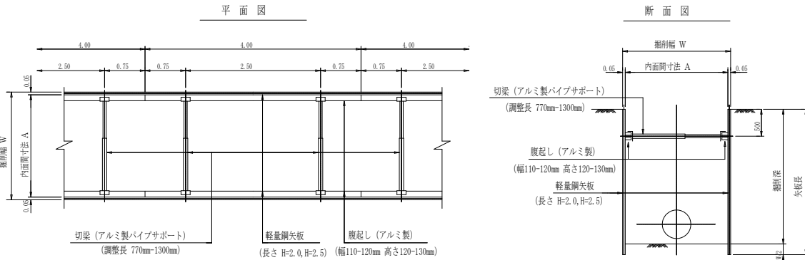
土留工 標準図 S=NON
