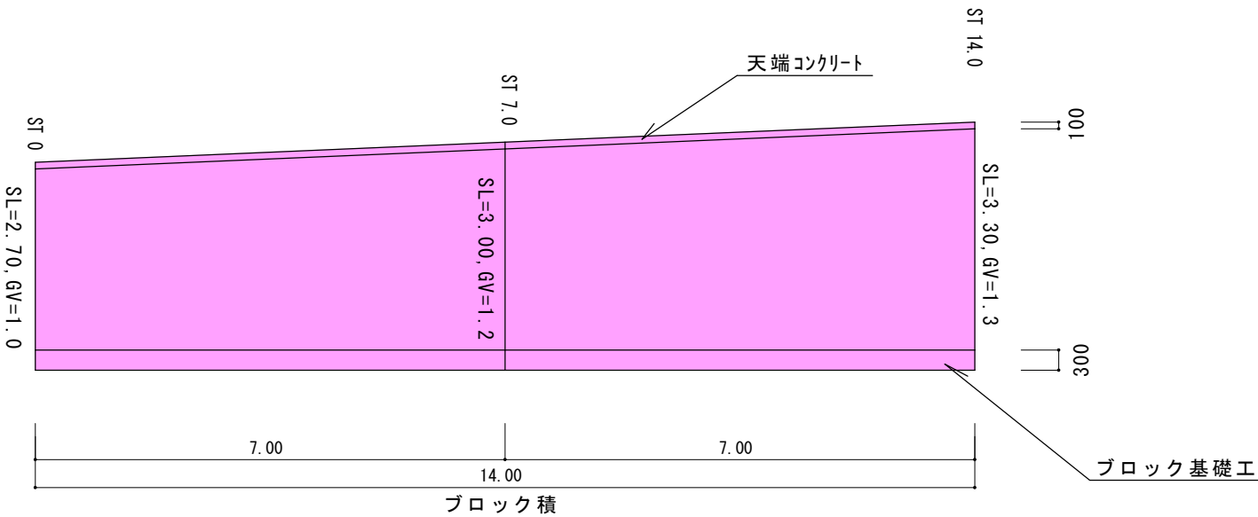
ブロック積展開図 S=1/100
