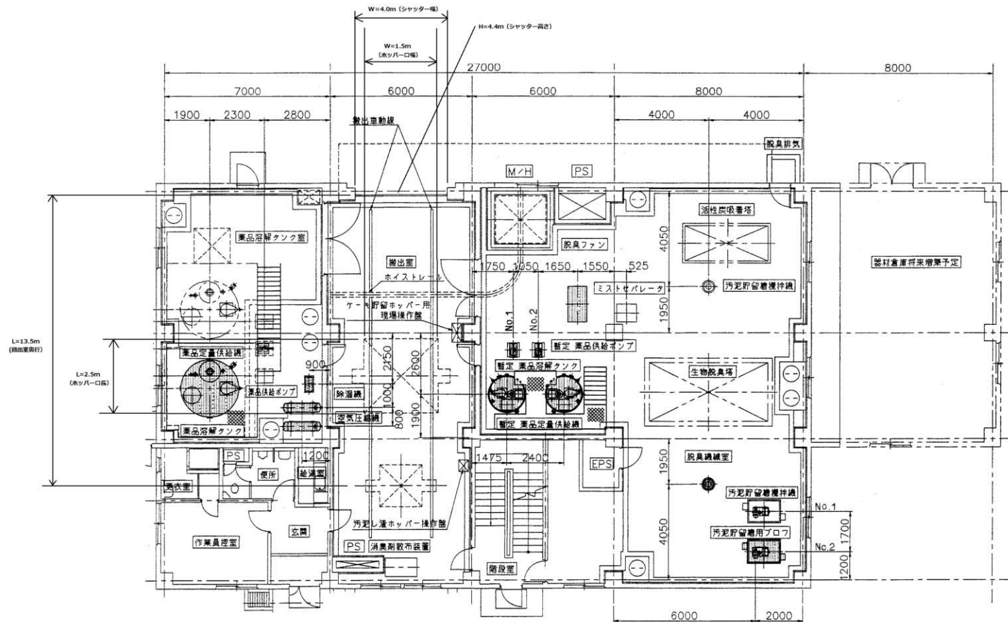
松永浄化センター汚泥処理棟 1 階平面図
