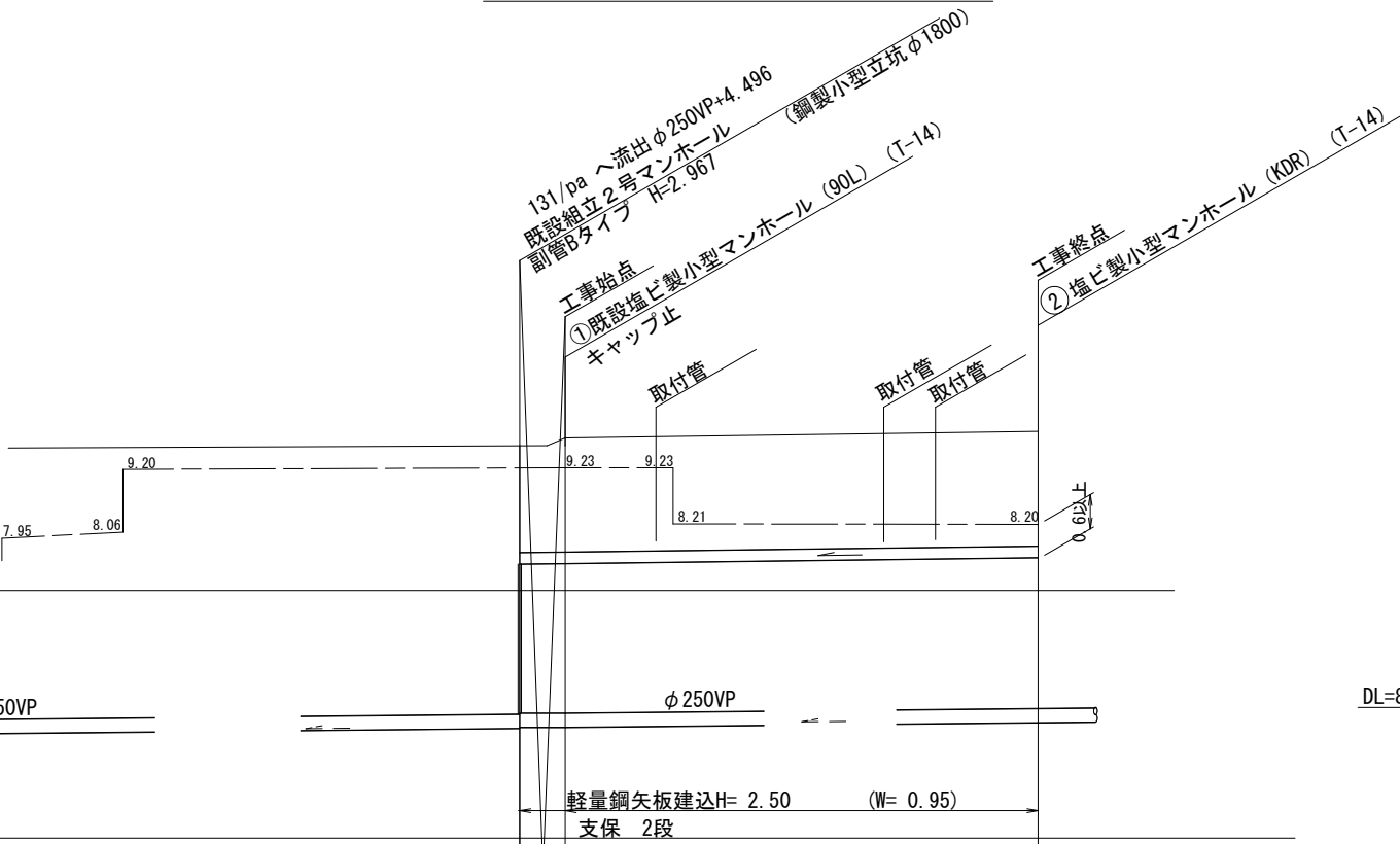
管渠埋設縦断面図 縦1/100 横1/500
