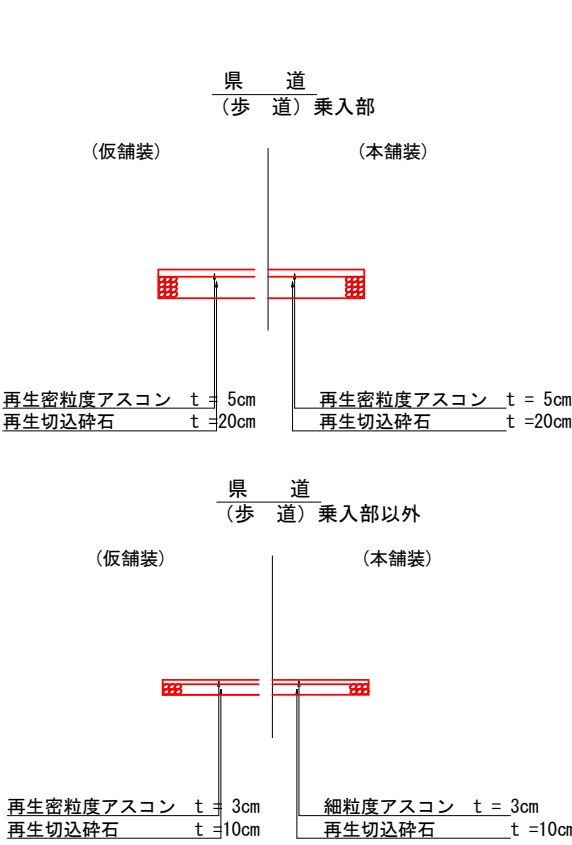
舗装断面図 S=1/10
