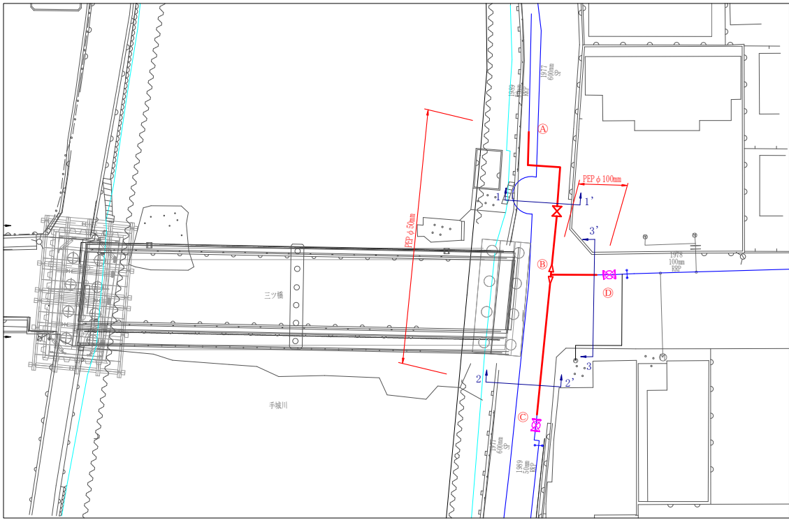
平面図 S=1/250
