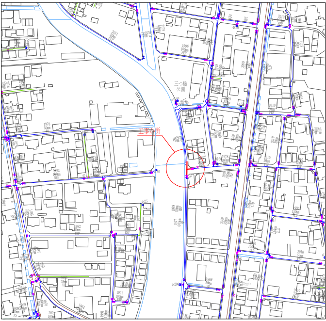
配管図 S=1/2500
