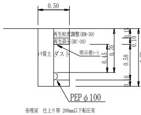
PEPφ100土工図
