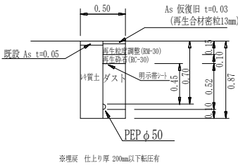
PEPφ50土工図①
