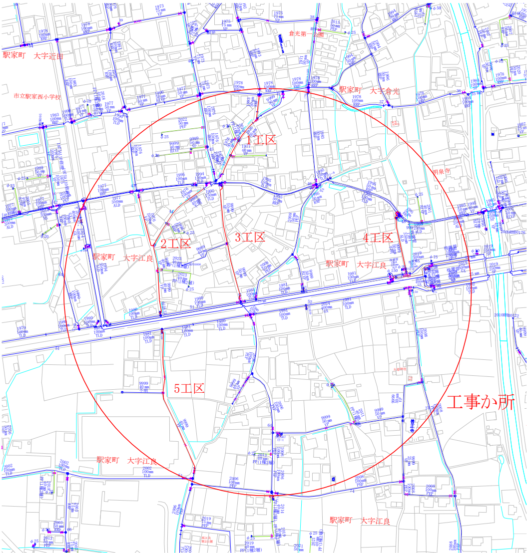
配管図
