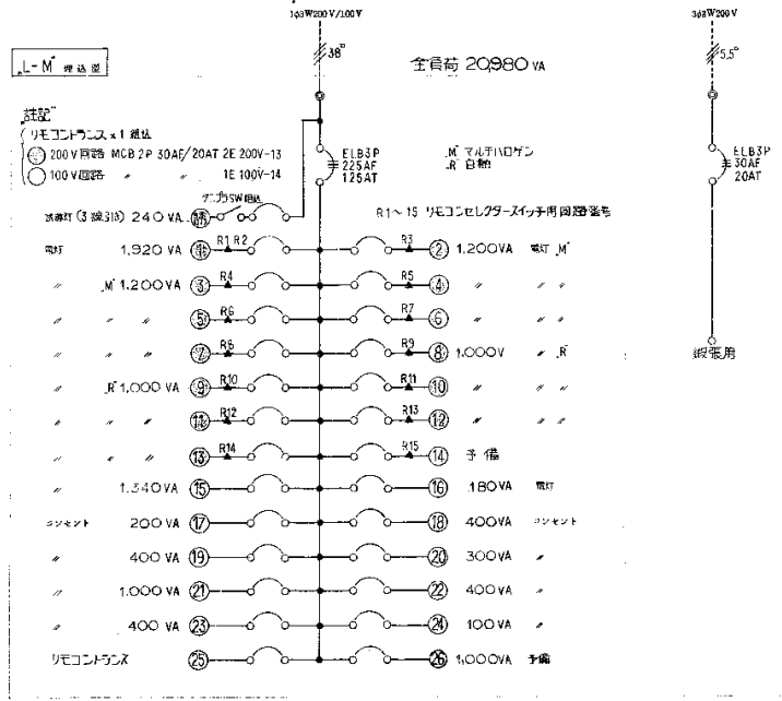
配分電盤結線図
