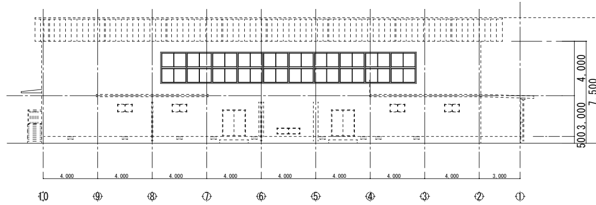
北立面図
