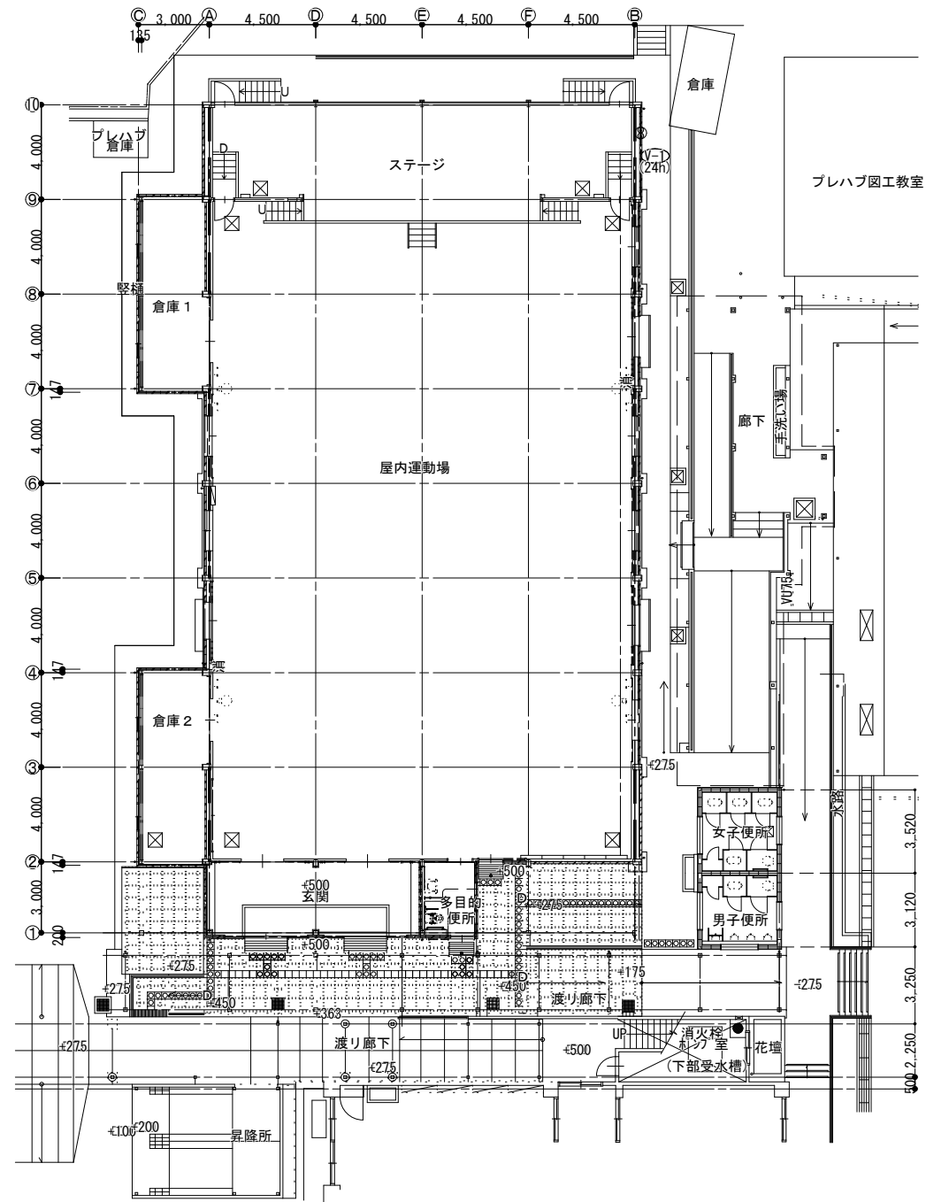
1階平面図 1:200
