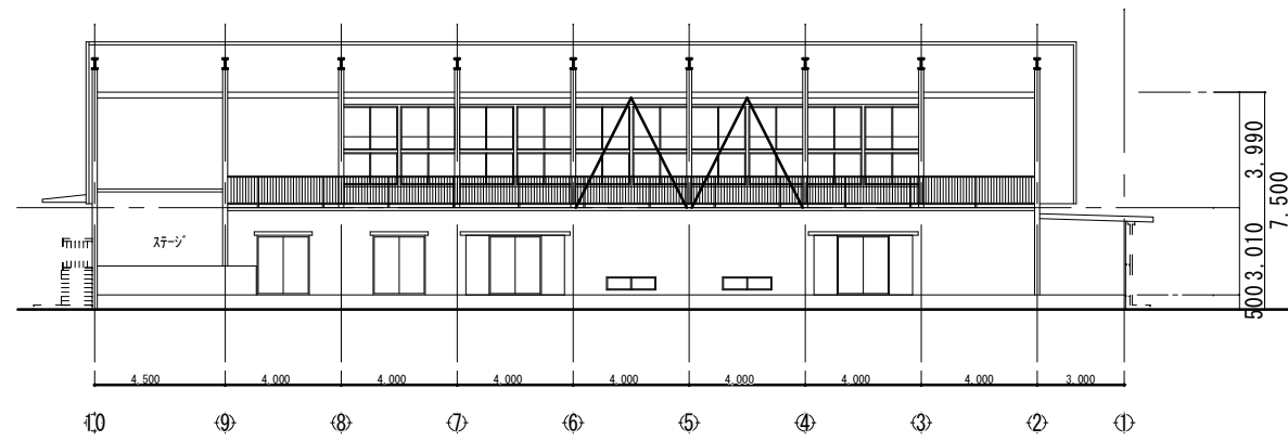
西展開図
