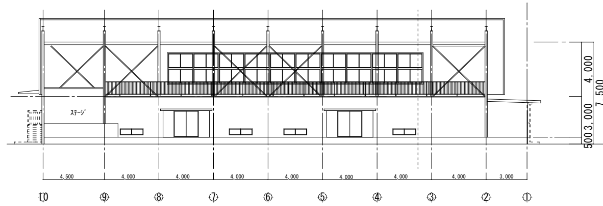
B 南展開図
