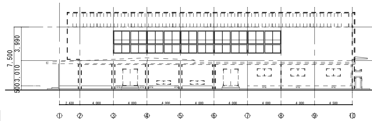
西立面図
