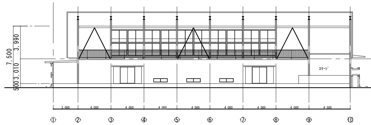
東展開図
