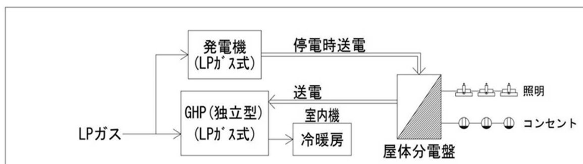
図1. 設備フロー図(熊野、津之郷小学校)
