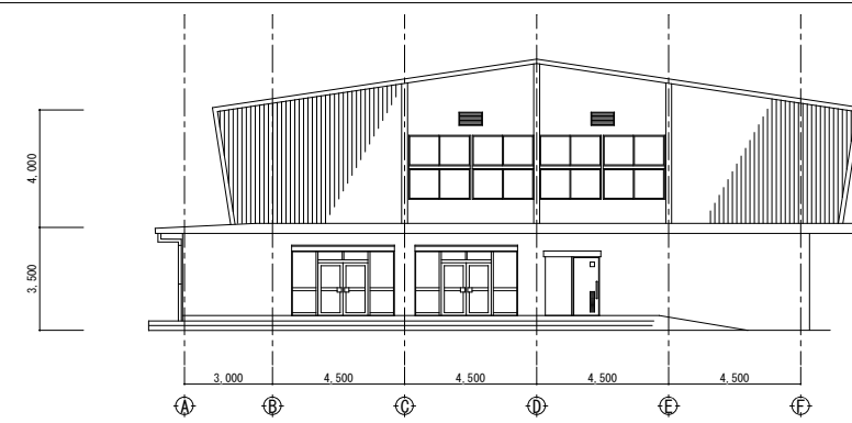
西側立面図 S=1:100
