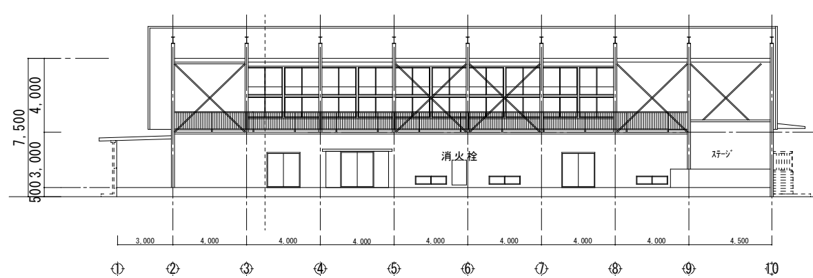
D 北展開図
