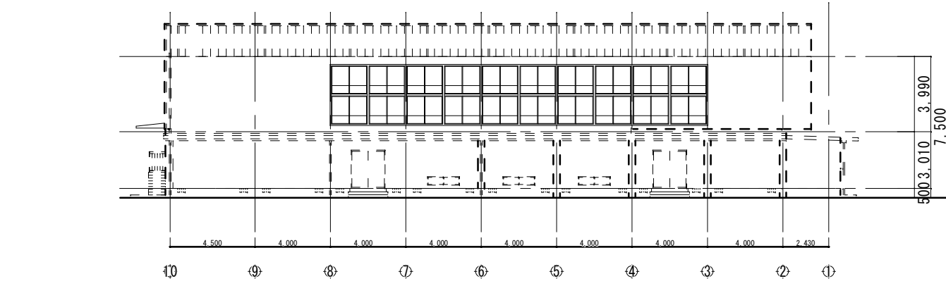
東立面図
