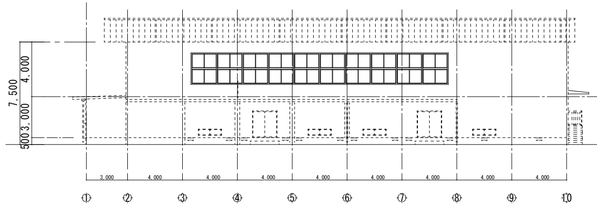
南立面図
