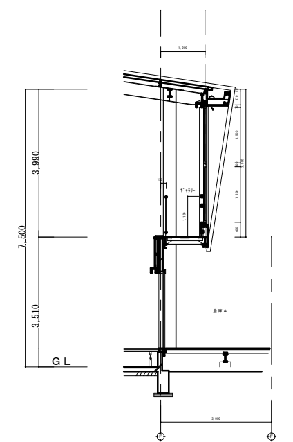
断面詳細図 1:100
