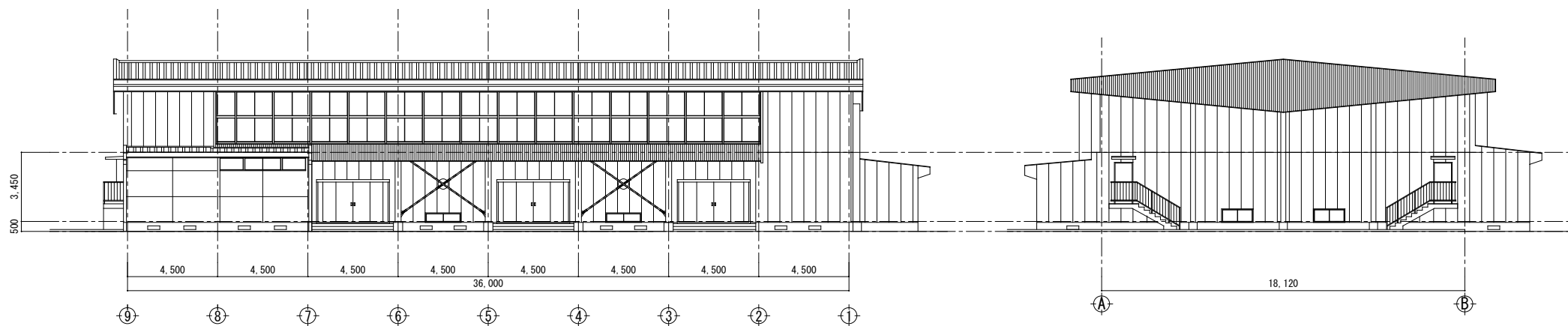
北側立面図
