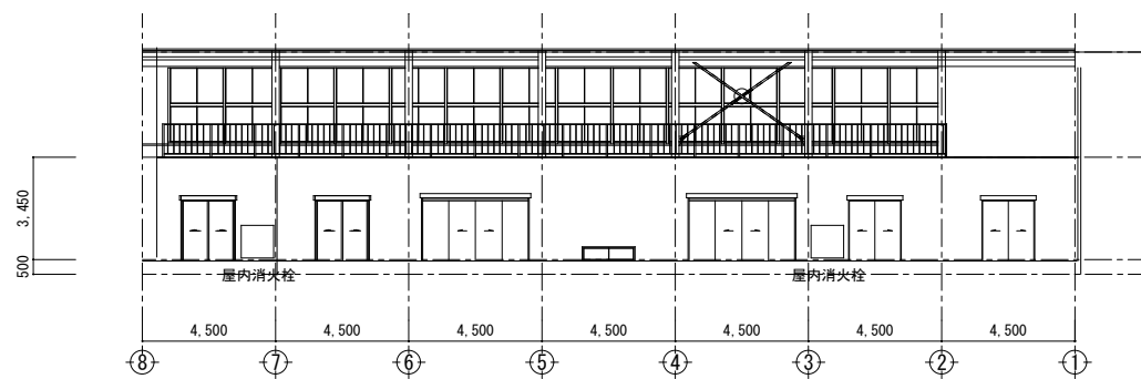
南面展開図
