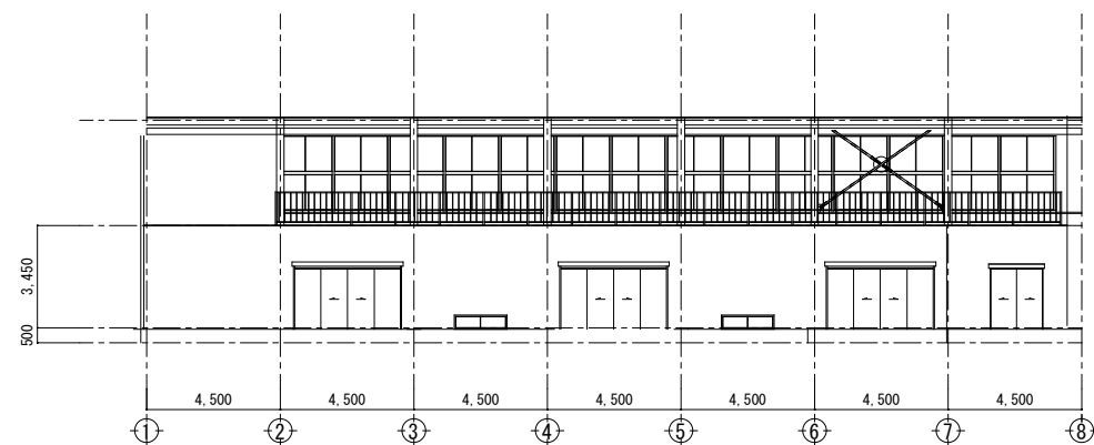
北面展開図
