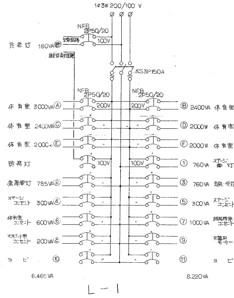
電灯分電盤
