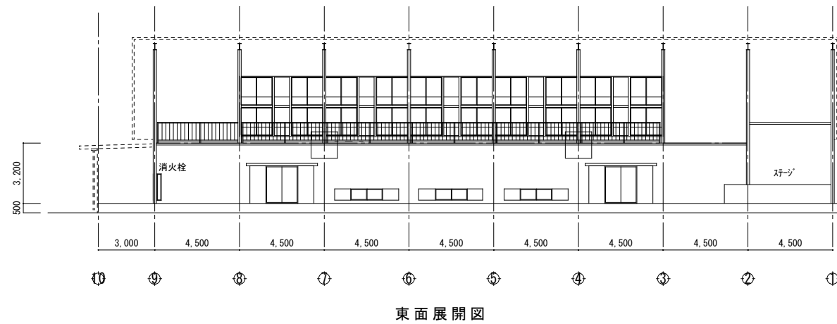
立面図 1:200
