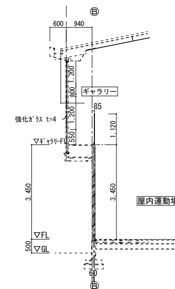
断面詳細 1:100
