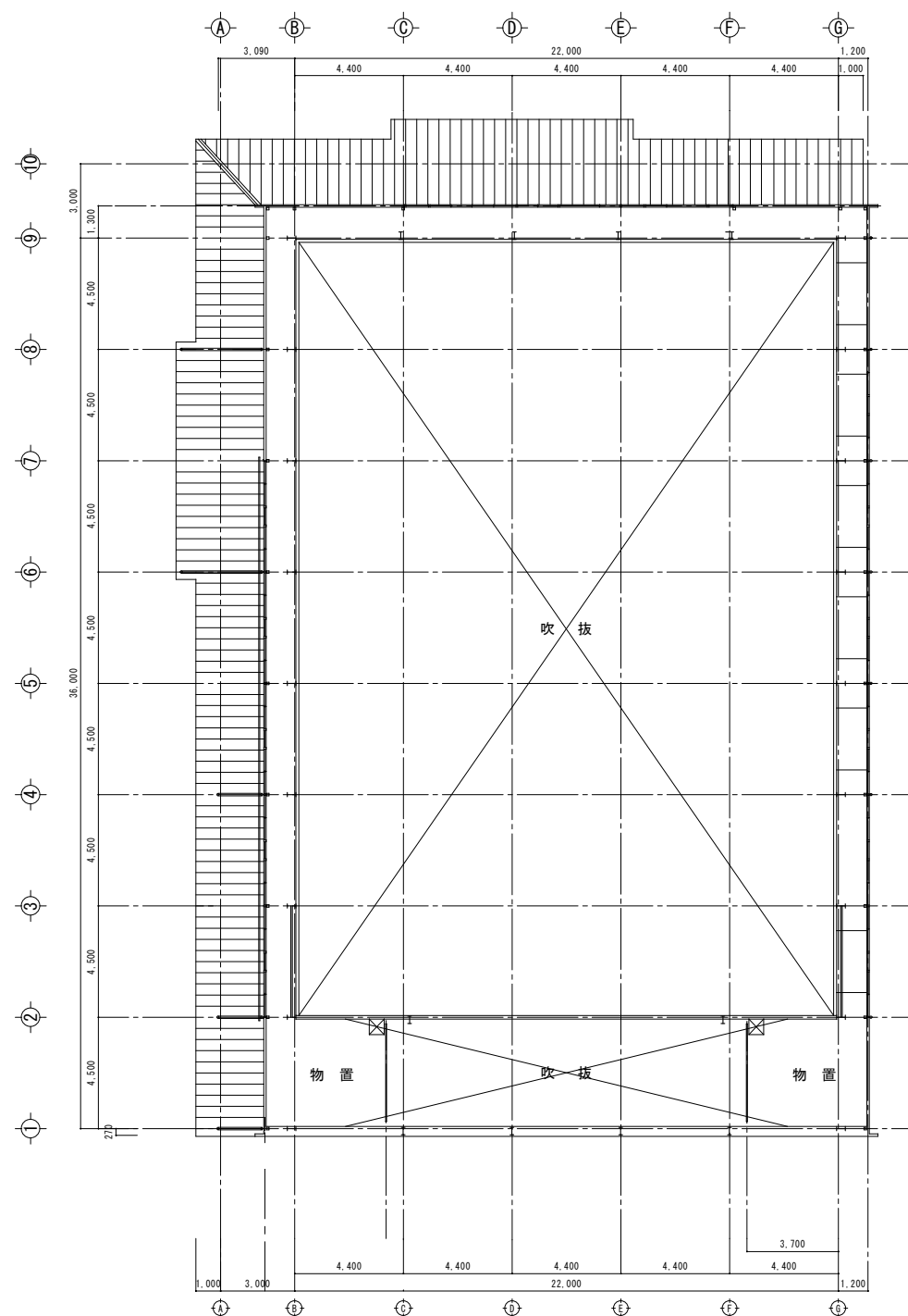
ギャラリー平面図 1:200
