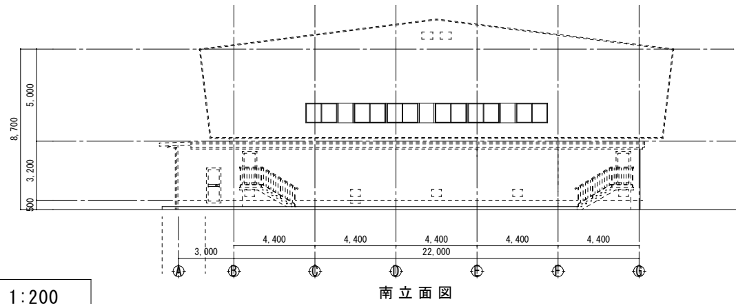
立面図 1:200
