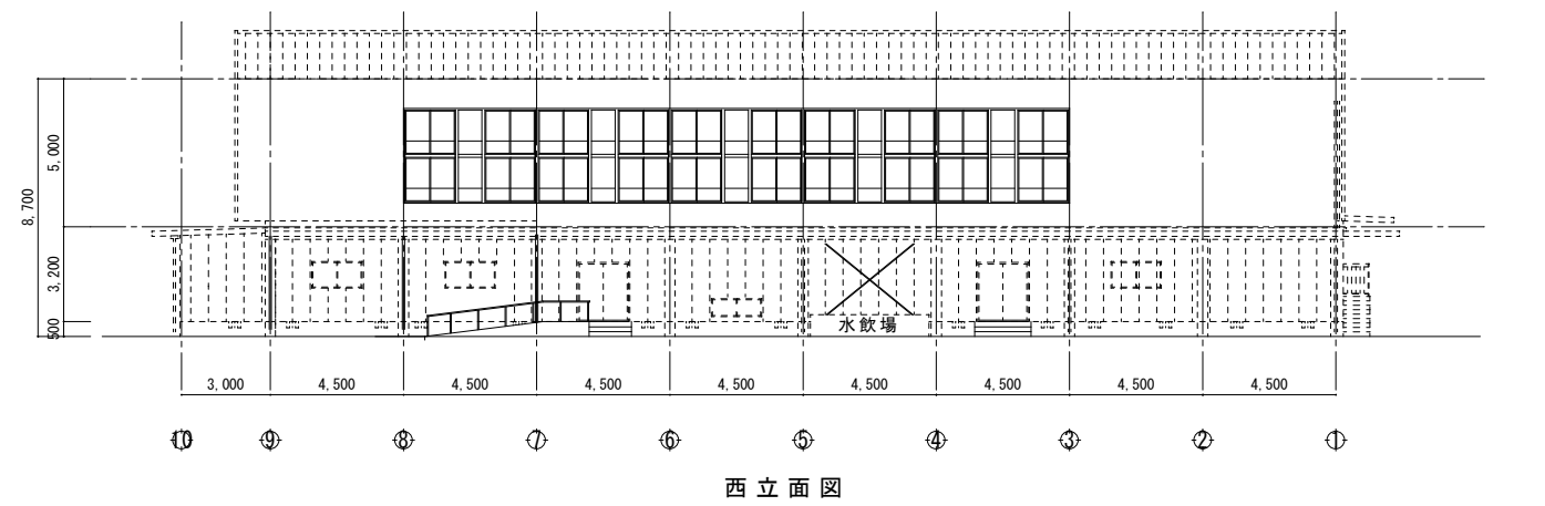
東立面図
