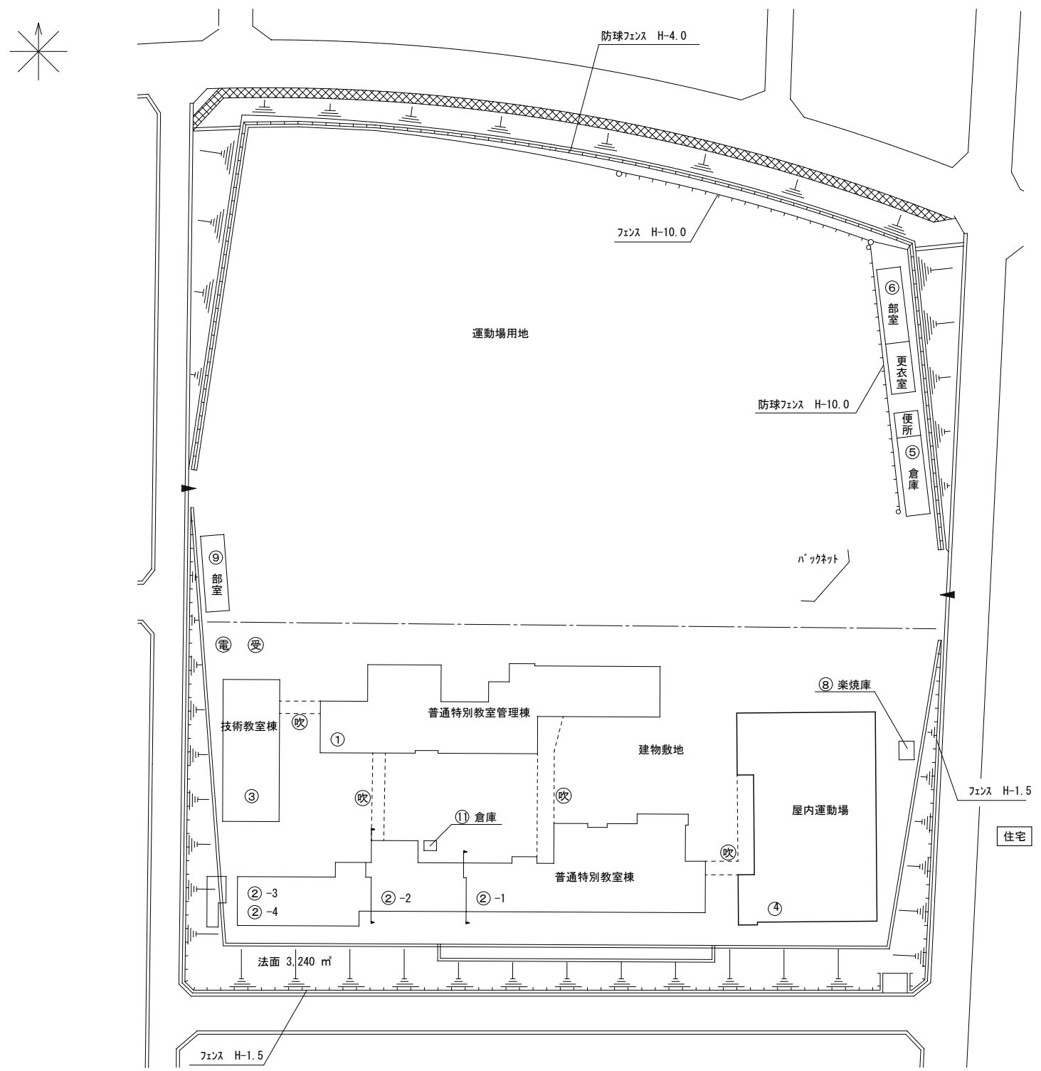
(東朋中学校) 配置図 1:700
