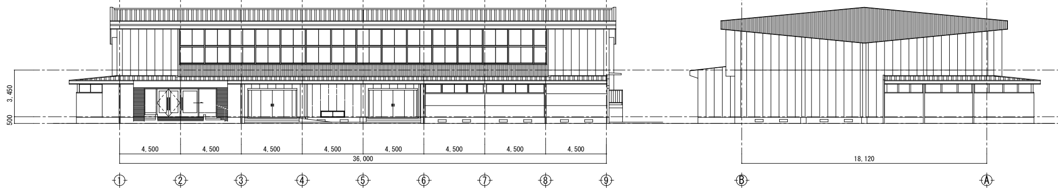
南側立面図
