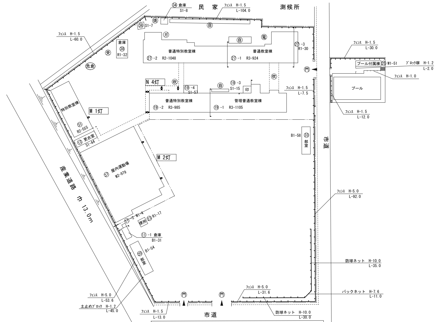
配置図 S=1/500
