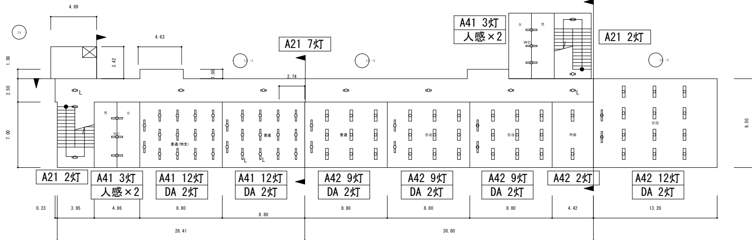
各階平面図 S=1/200
