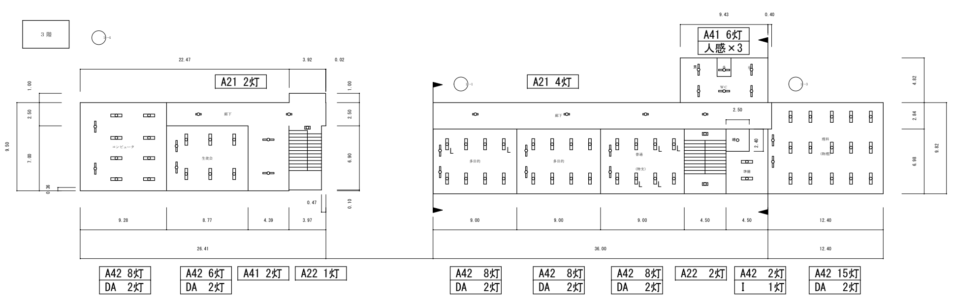
各階平面図 S=1/200
