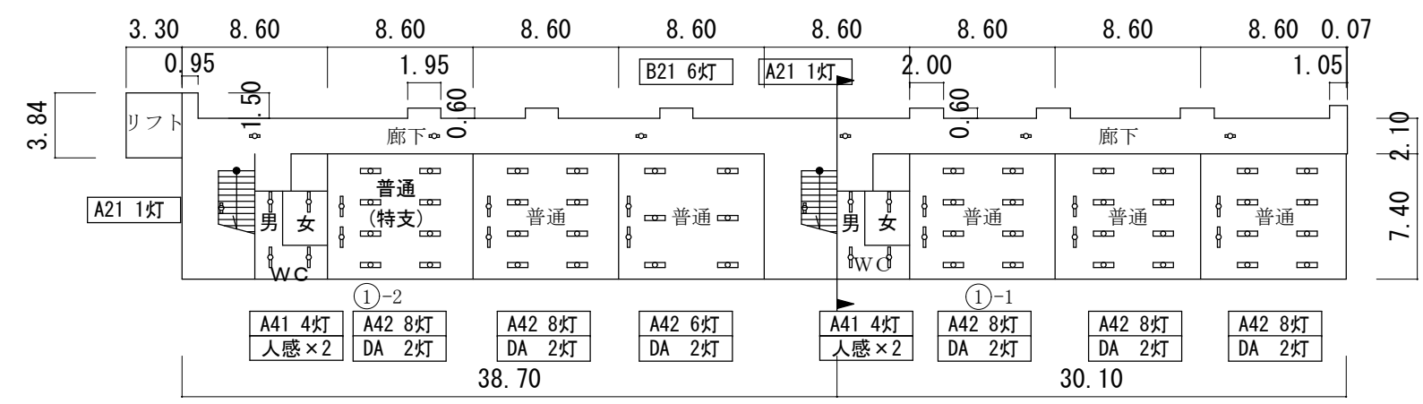
各階平面図 S=1/200
