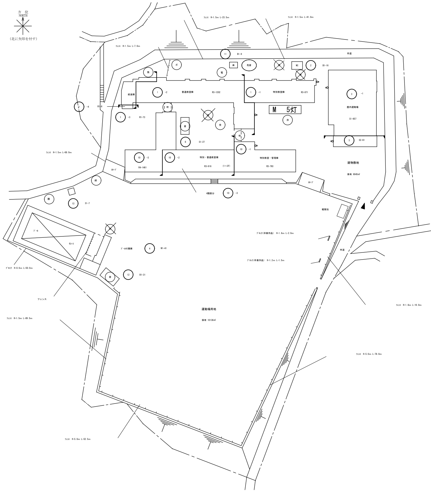
配置図 S=1/500
