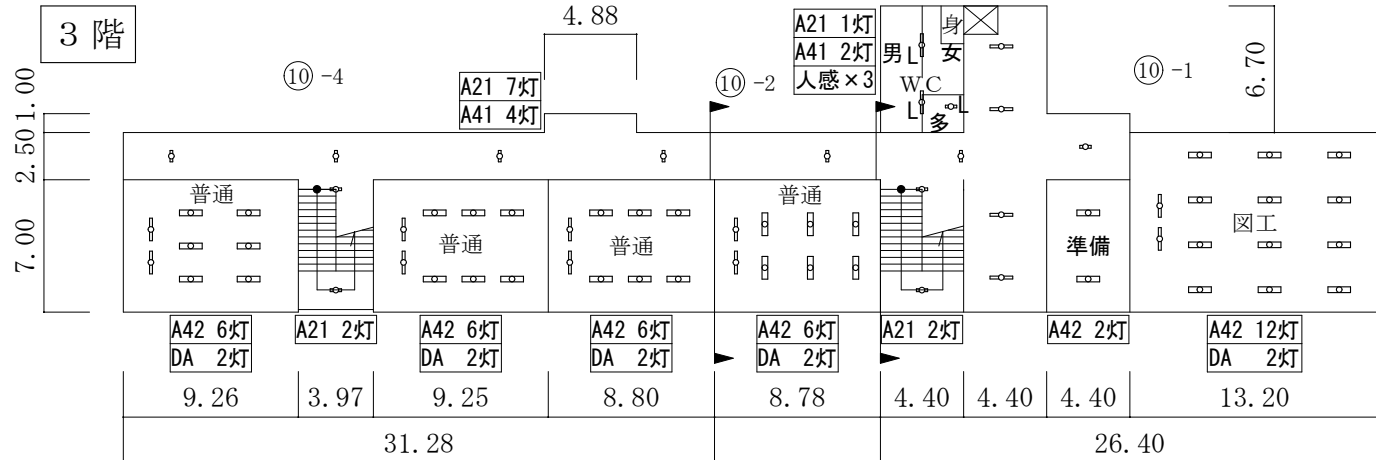
各階平面図 S=1/200
