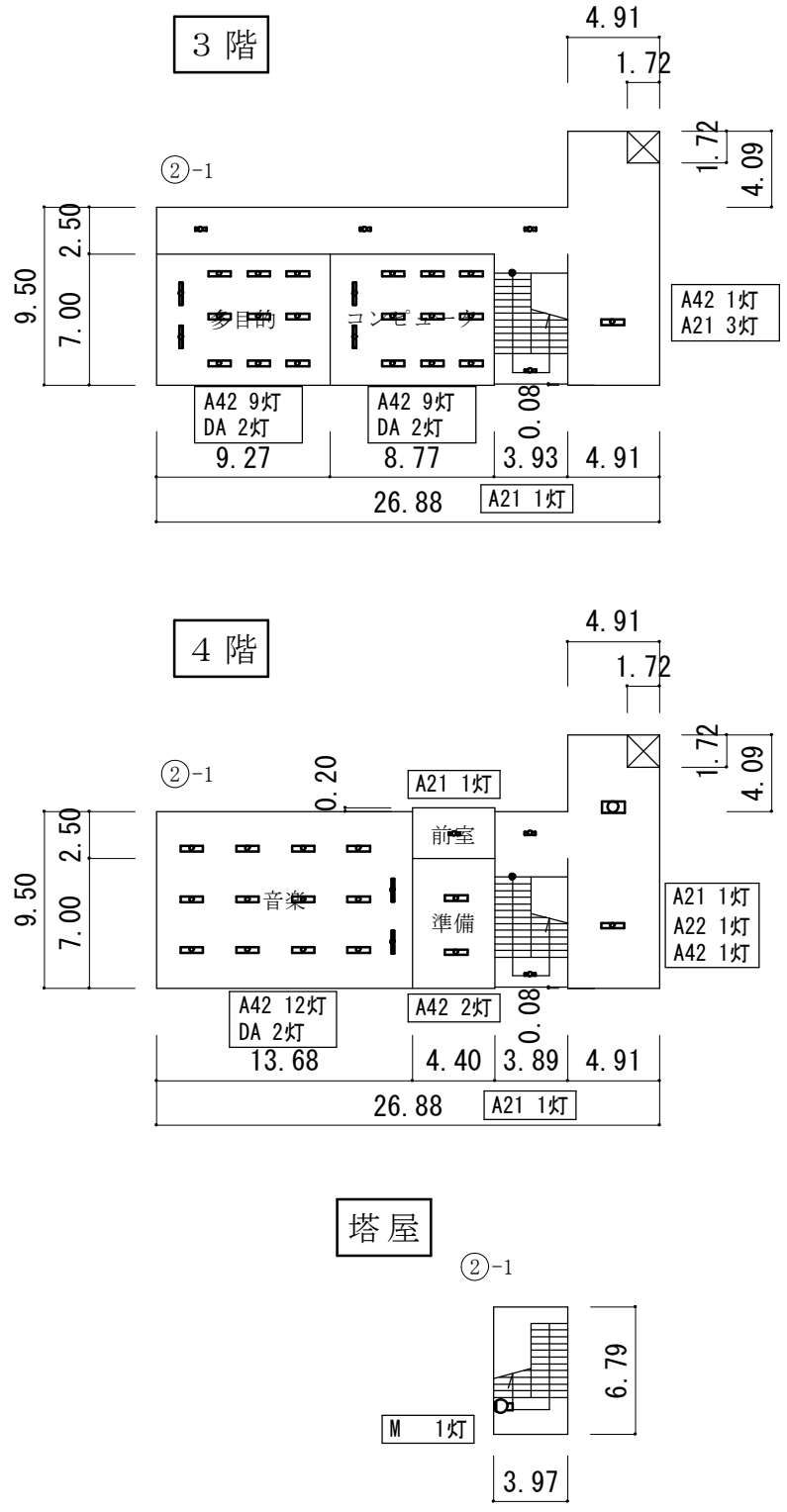
各階平面図 S=1/200
