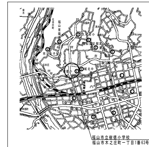
付近見取図
