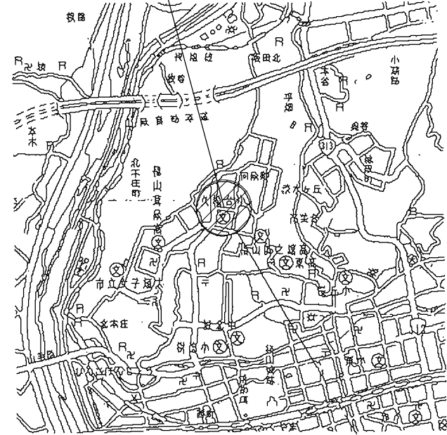
付近見取図
