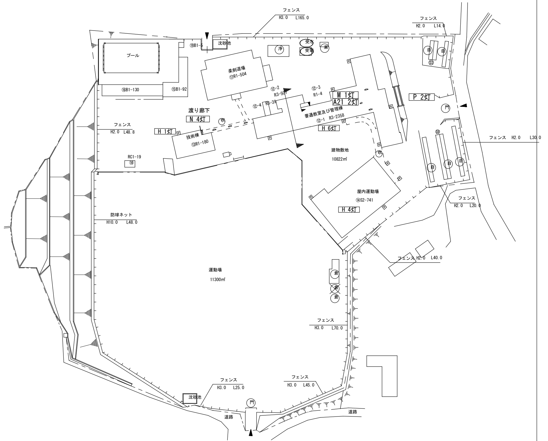
配置図 S=1/500
