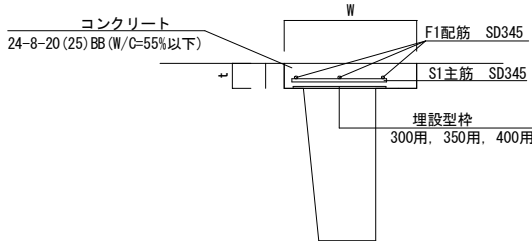
撤去しない埋設型枠 S=1:40
