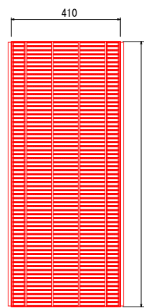
コンクリート蓋、グレーチング蓋 S=1:20 落ちふた式U型側溝3種ふた300 ノンスリップかさがあげ、T-25、細目ゴム付
