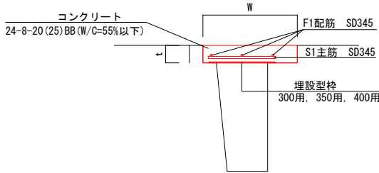
撤去しない埋設型枠 S=1:40
