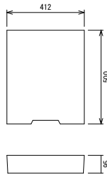
コンクリート蓋、グレーチング蓋 S=1:20 落ちふた式U型側溝3種ふた300 ノンスリップかきあげ、T-25、細目ゴム付
