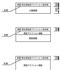
舗装標準断面図 S=1:20
