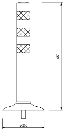
車線分離標 S=1:10
