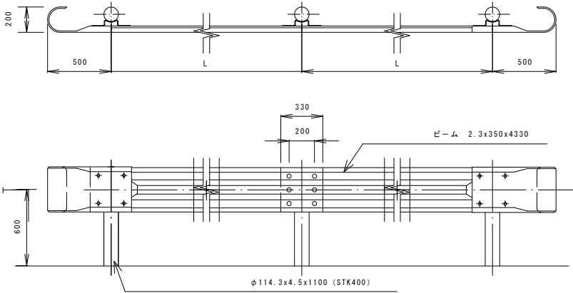
平面・正面図
