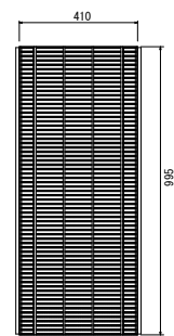
コンクリート蓋、グレーチング蓋 S=1:20 落ちふた式U型側溝3種ふた300 ノンスリップかきあげ、T-25、細目ゴム付
