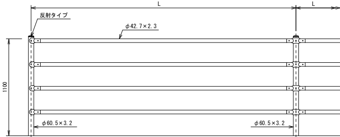
転落防止柵(P種)
