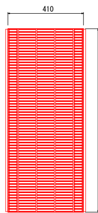
コンクリート蓋、グレーチング蓋 S=1:20 落ちふた式U型側溝3種ふた300 ノンスリップかさあげ、T-25、細目ゴム付
