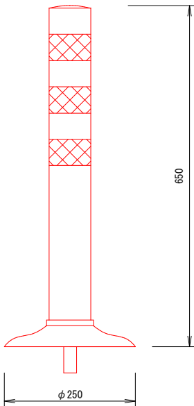
車線分離標 S=1:10
