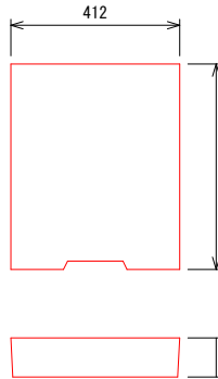
コンクリート蓋、グレーチング蓋 S=1:20 落ちふた式U型側溝3種ふた300 ノンスリップかさあげ、T-25、細目ゴム付
